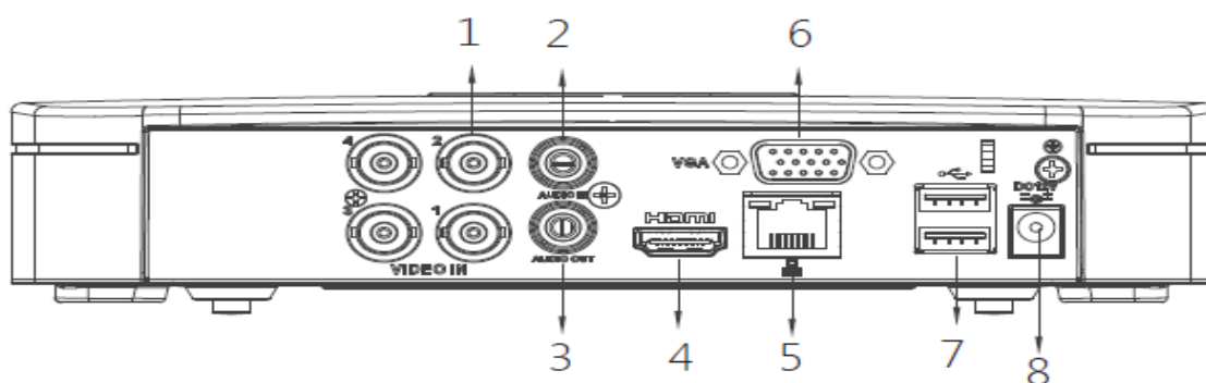
Рисунок 2 Внешний вид задней панели.
