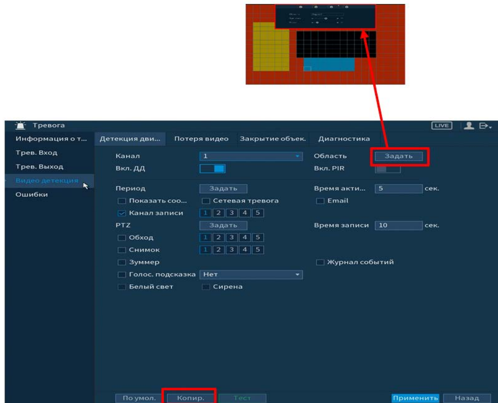
Рисунок 6.18 – Настройка области
