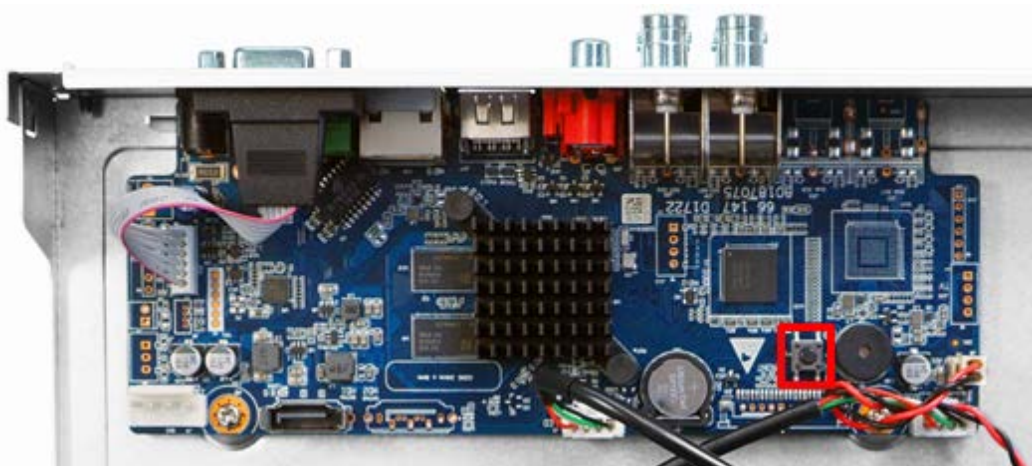
Рисунок 7.10 – Кнопка сброса
