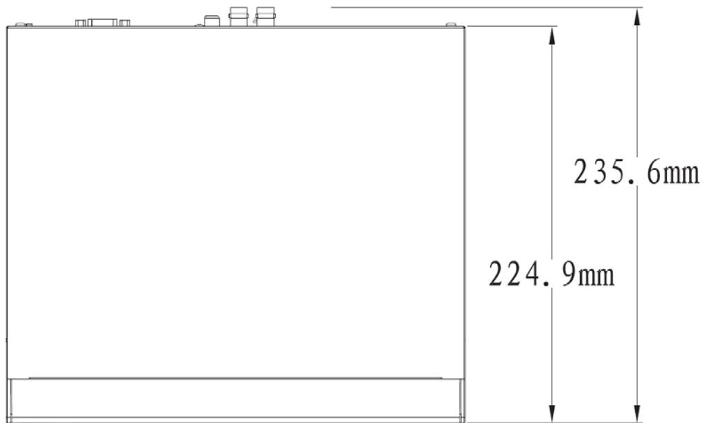
Рисунок 3.9 – Габаритные размеры видеореєстратора
