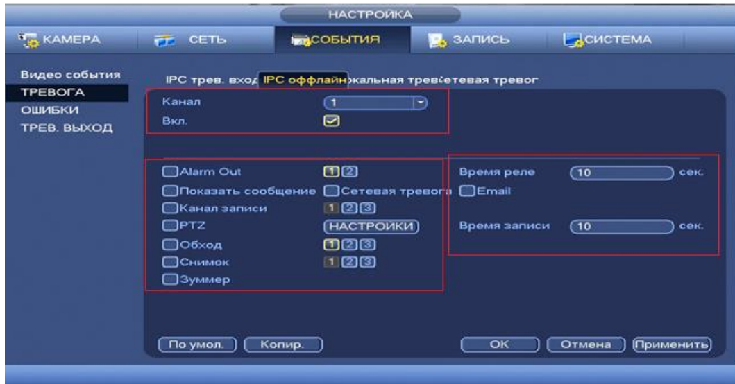
Рисунок 8.84 Интерфейс настройки IPС-оффлайн.
