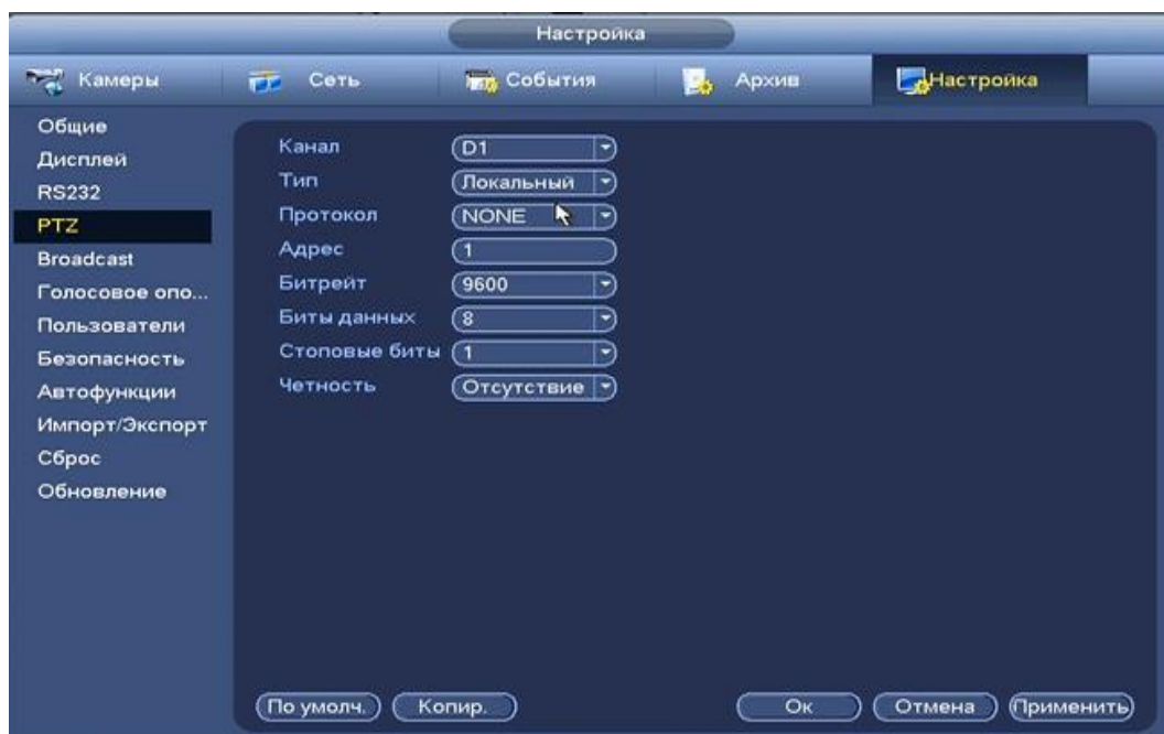
Рисунок 8.127 Интерфейс настройки при локальном типе.
