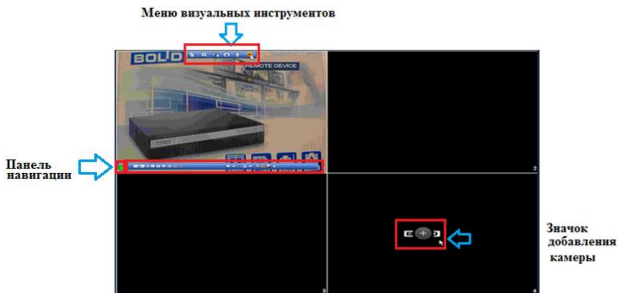
Рисунок 7.3 Добавление IP-камер.
