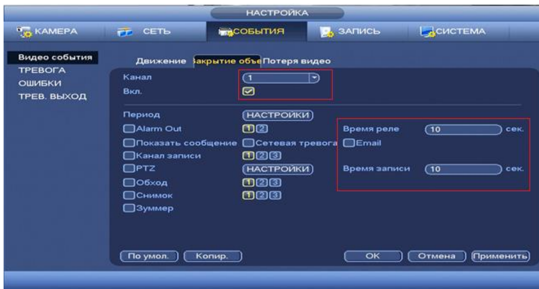
Рисунок 8.75 Установка настроек.
