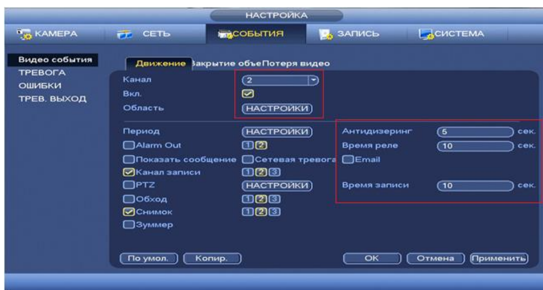
Рисунок 8.64 Установка настроек
