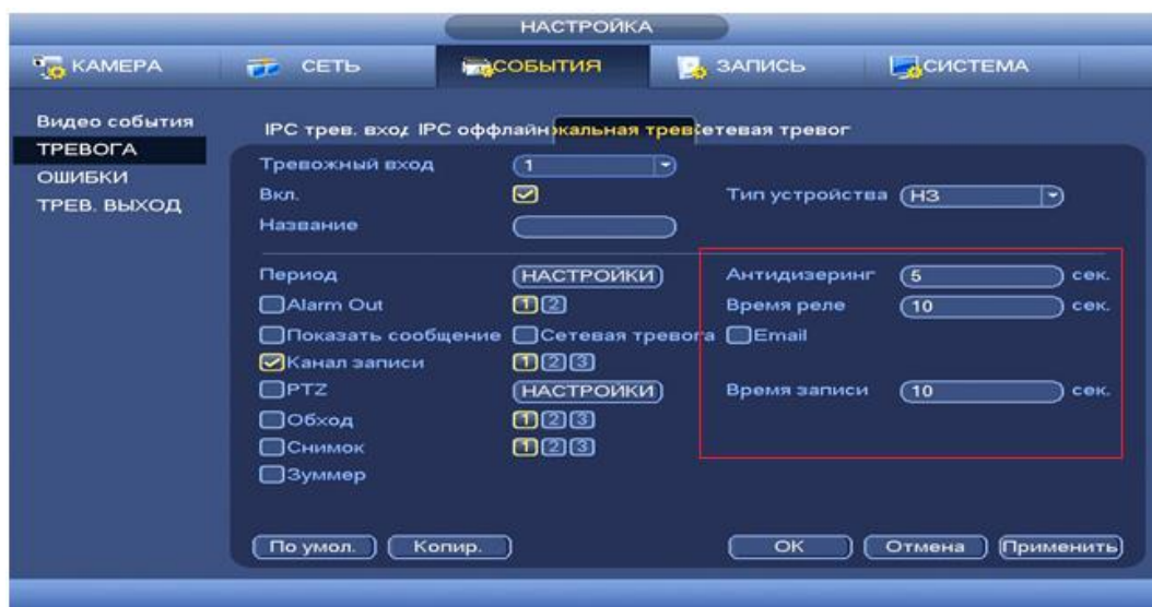
Рисунок 8.91 Установка настроек.
