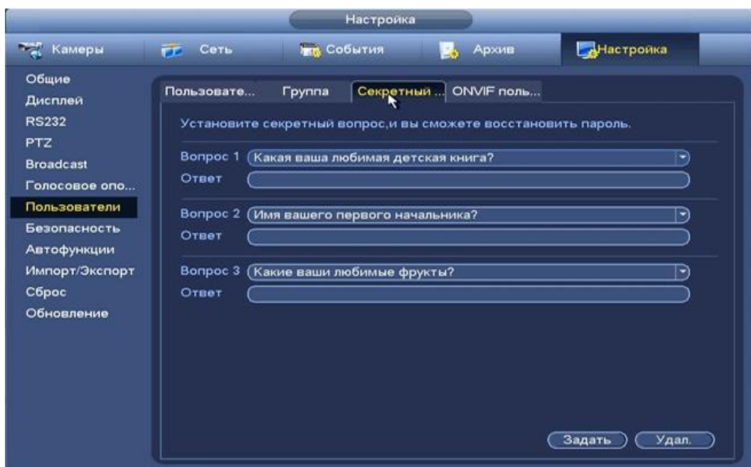
Рисунок 8.133 Интерфейс настройки
