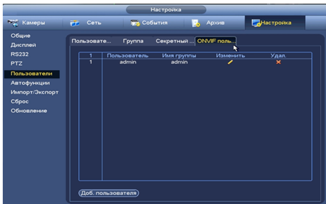
Рисунок 8.134 Настройка ONVIF.
