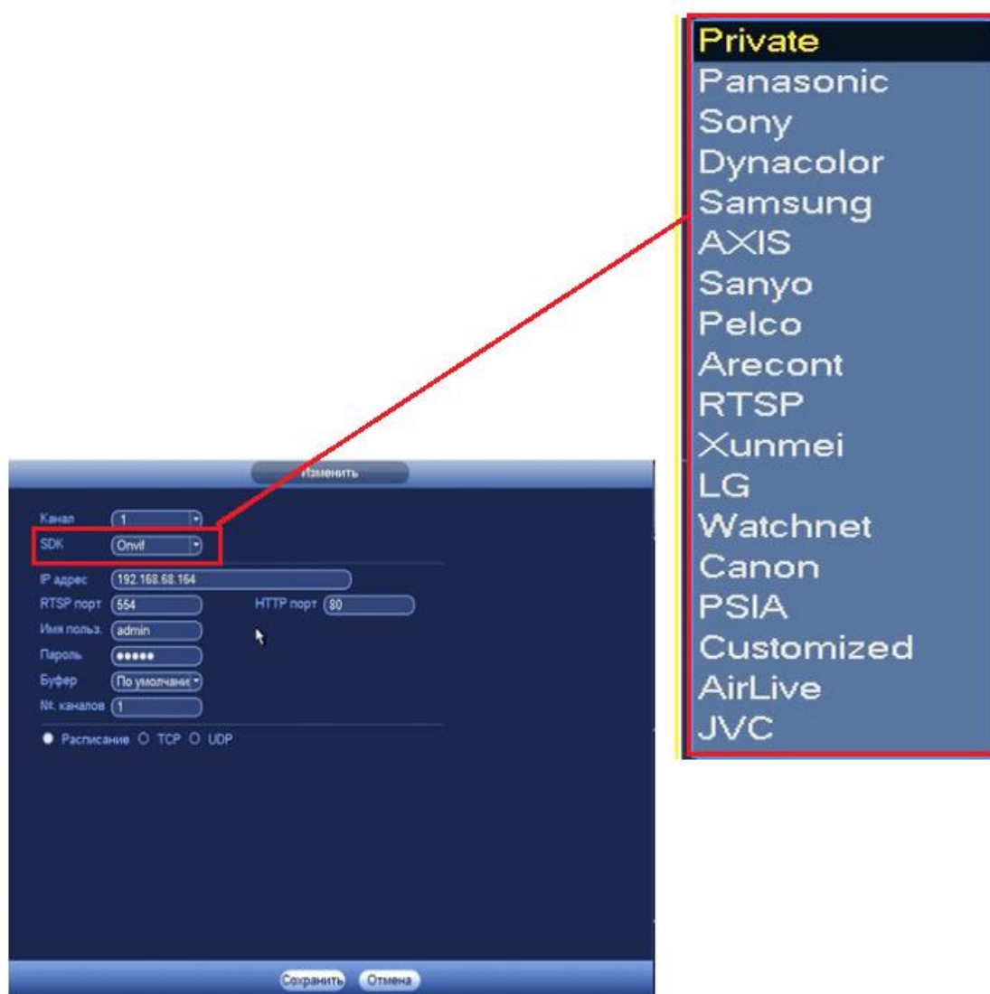
Рисунок 6.9 Настройка добавления камер сторонних производителей.
