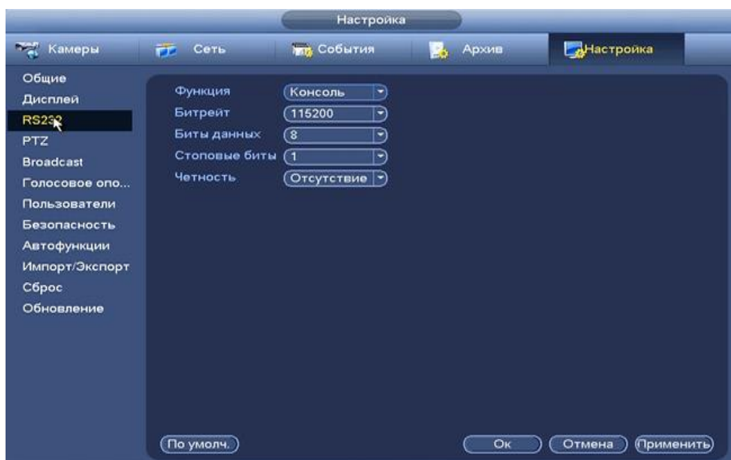
Рисунок 8.125 Интерфейс настройки
