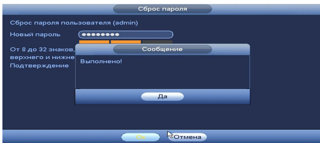
Рисунок 8.147 Ввод пароля.
