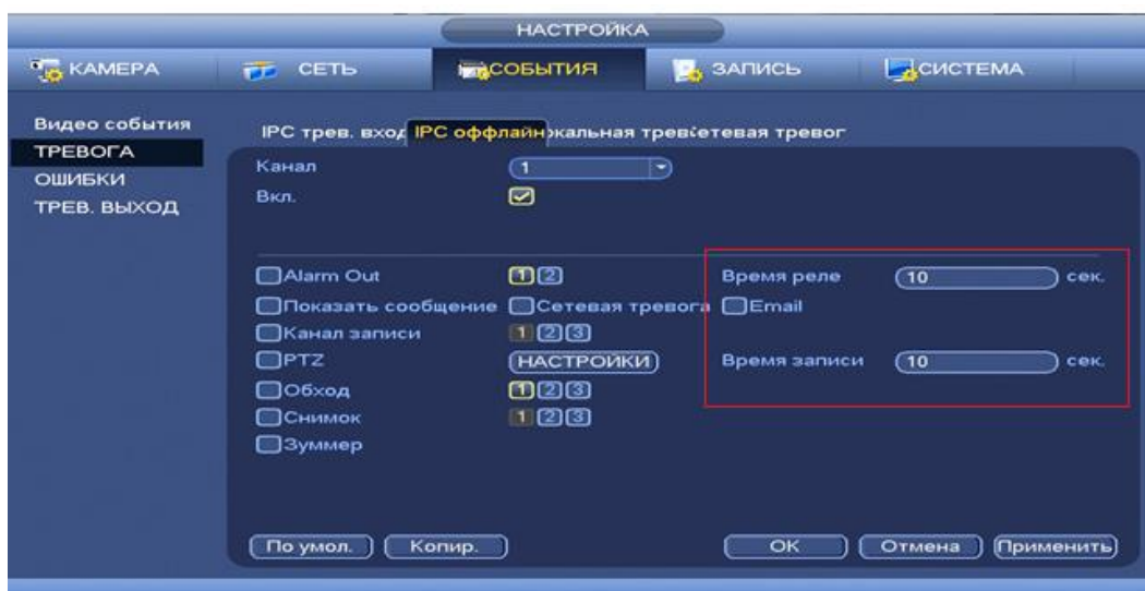
Рисунок 8.85 Установка настроек
