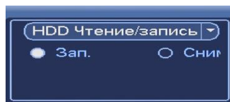
Рисунок 8.5 Тип поиска
