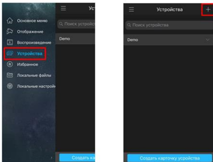
Рисунок 9.3 Меню устройства
