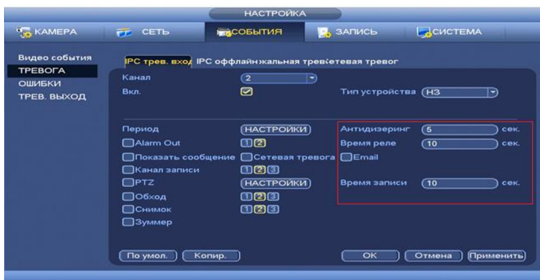
Рисунок 8.81 Установка настроек.
