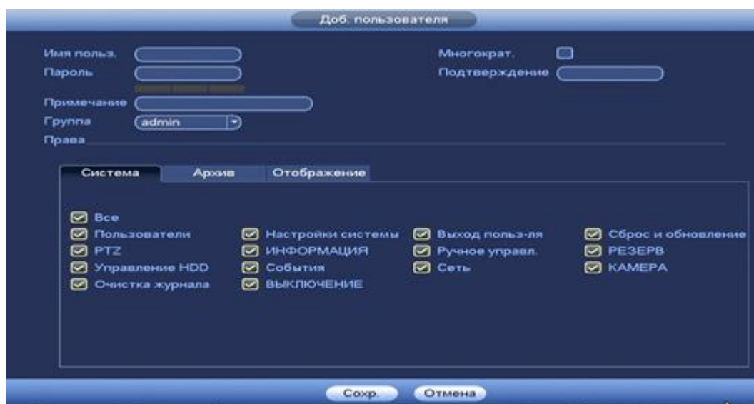
Рисунок 8.130 Добавление пользователя.
