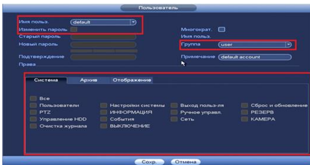
Рисунок 8.129 Назначение прав.
