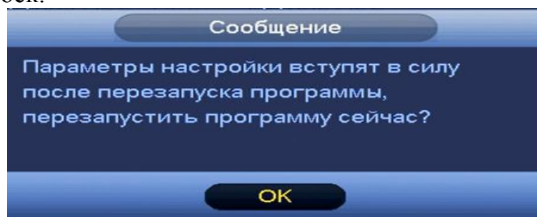
Рисунок 8.114 Всплывающее сообщение.
