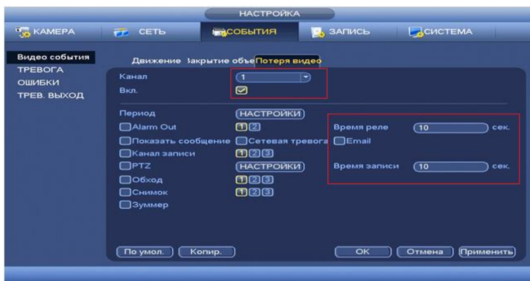
Рисунок 8.70 Установка настроек.
