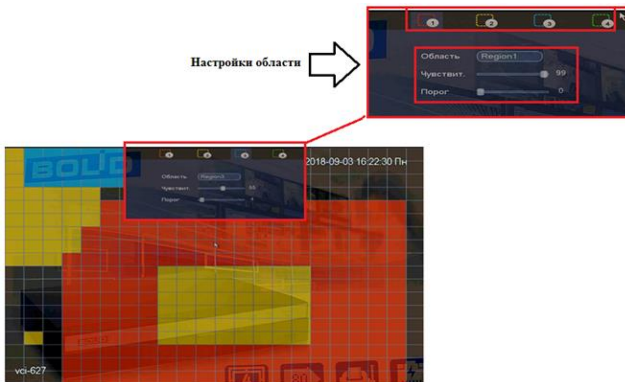
Рисунок 8.60 Настройка области.
