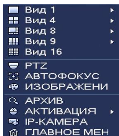
Рисунок 7.1 Контекстное меню.
