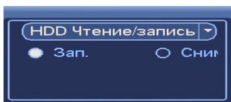
Рисунок 7.17 Тип поиска.
