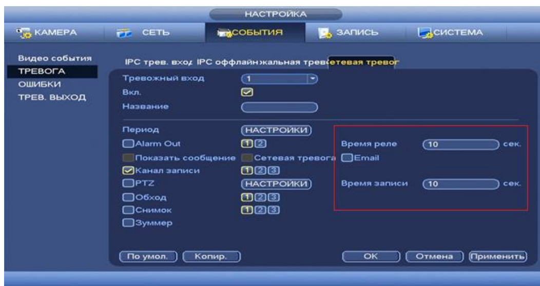
Рисунок 8.97 Установка настроек.
