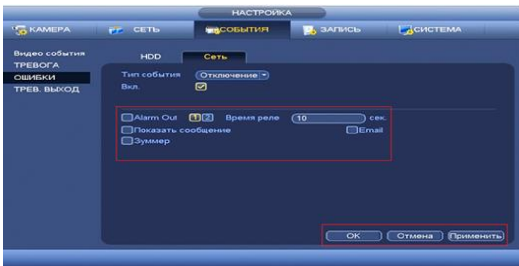
Рисунок 8.102 Установка настроек.
