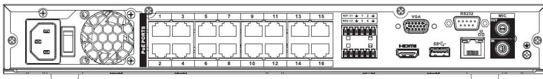
Рисунок 2 Задняя панель.
