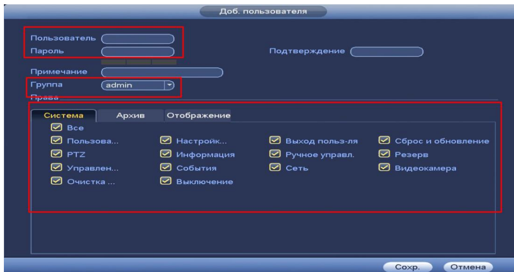
Рисунок 8.132 Назначение прав.
