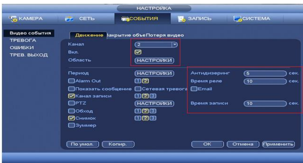
Рисунок 8.65 Установка настроек
