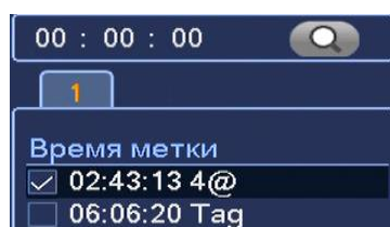
Рисунок 7.22 Выбор метки.
