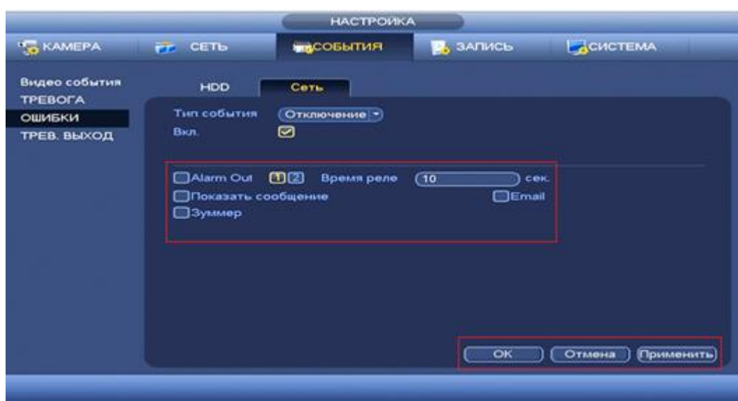
Рисунок 8.104 Установка настроек.
