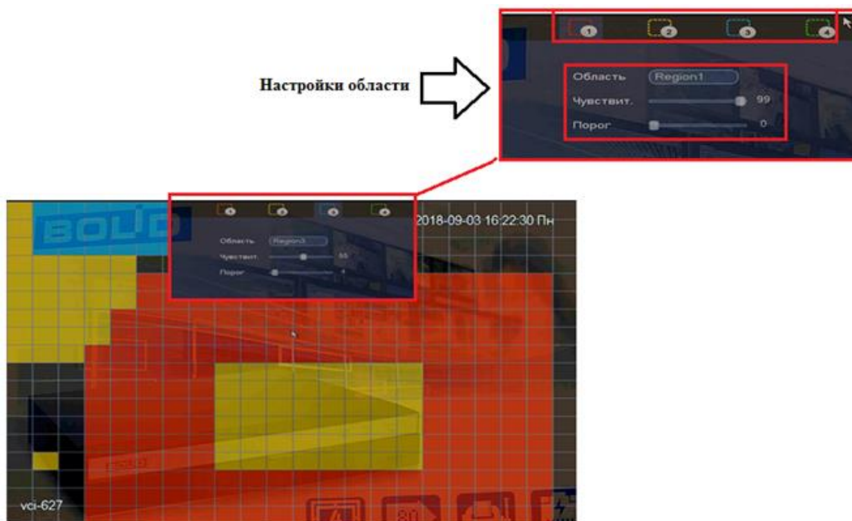
Рисунок 8.61 Настройка области.
