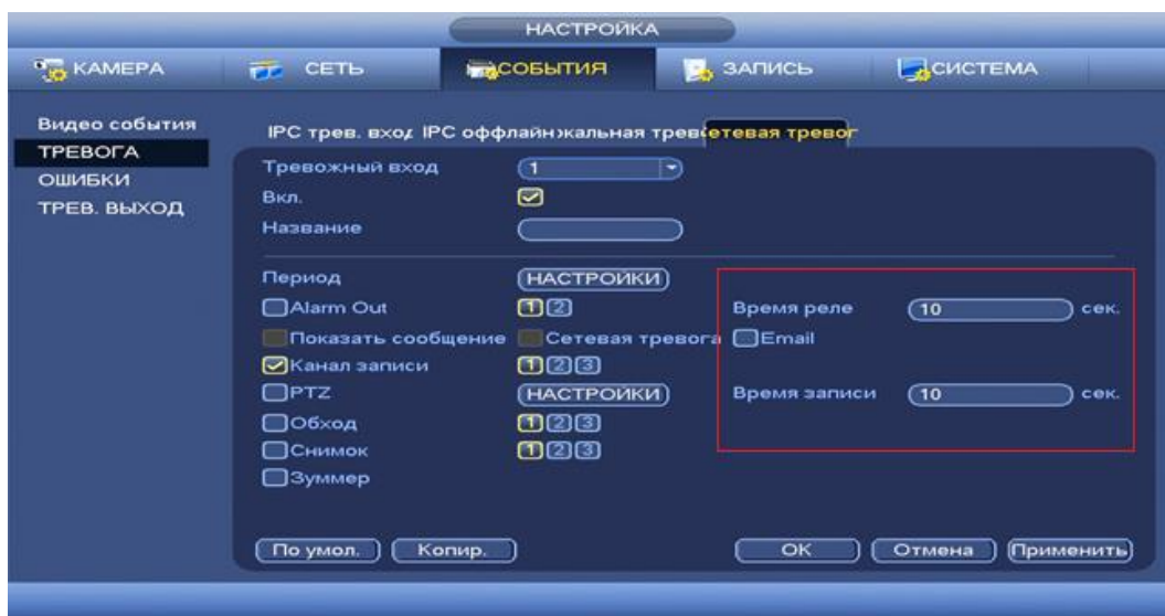
Рисунок 8.99 Установка настроек.
