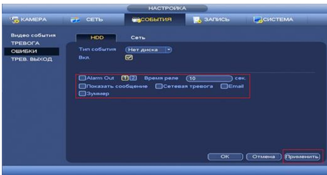
Рисунок 8.102 Установка настроек.
