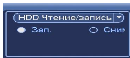
Рисунок 8.5 Тип поиска
