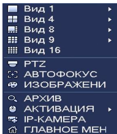
Рисунок 7.1 Контекстное меню.
