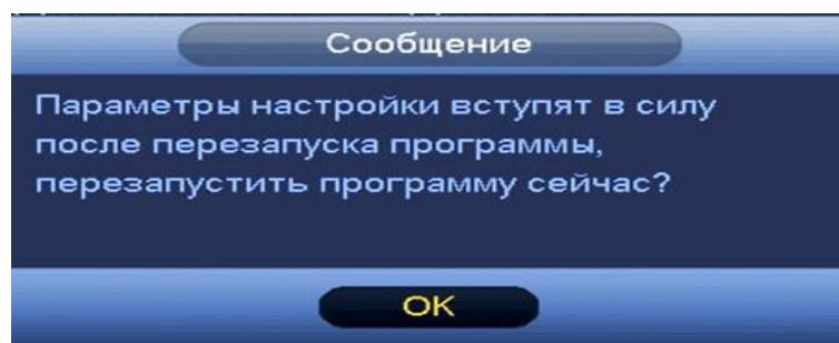
Рисунок 8.117 Всплывающее сообщение.
