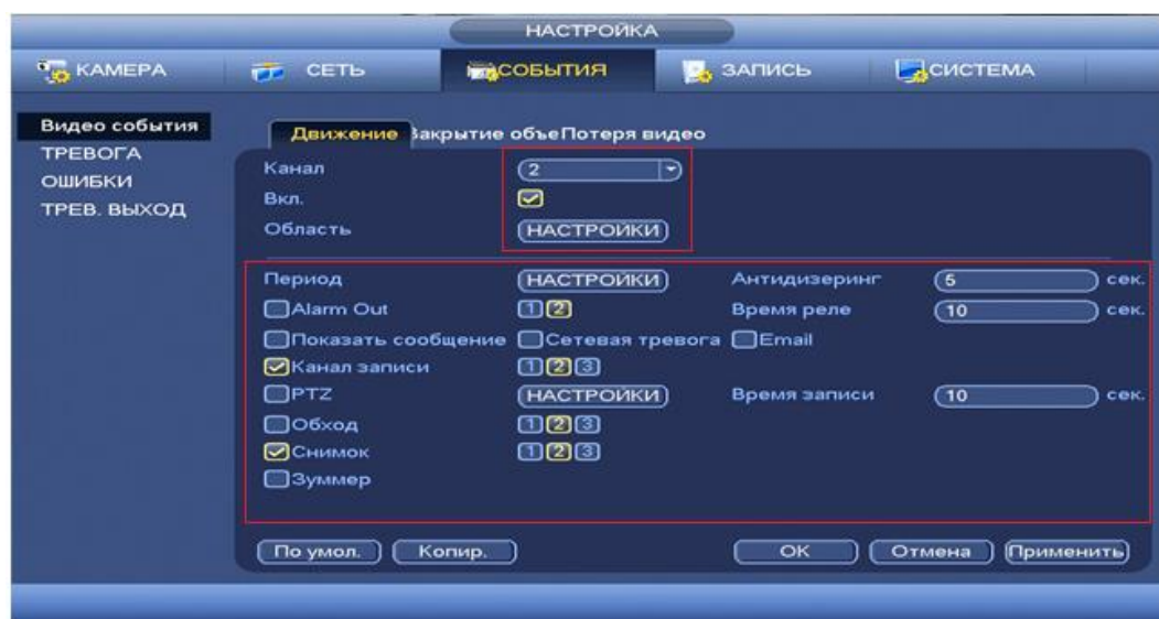
Рисунок 8.60 Настройка события
