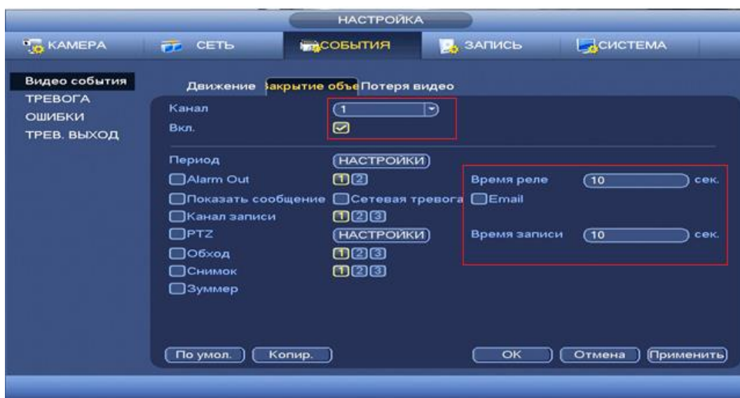
Рисунок 8.71 Установка настроек.
