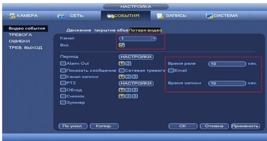
Рисунок 8.77 Установка настроек.
