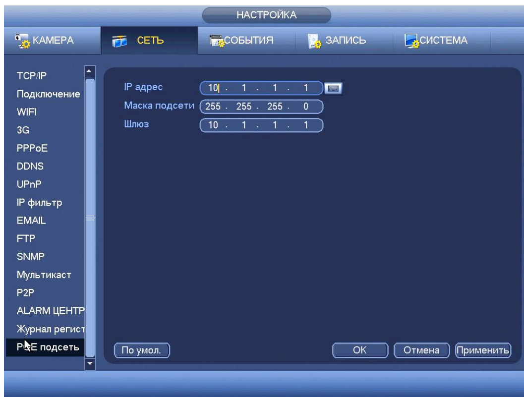
Рисунок 8.59 Интерфейс настройки.
