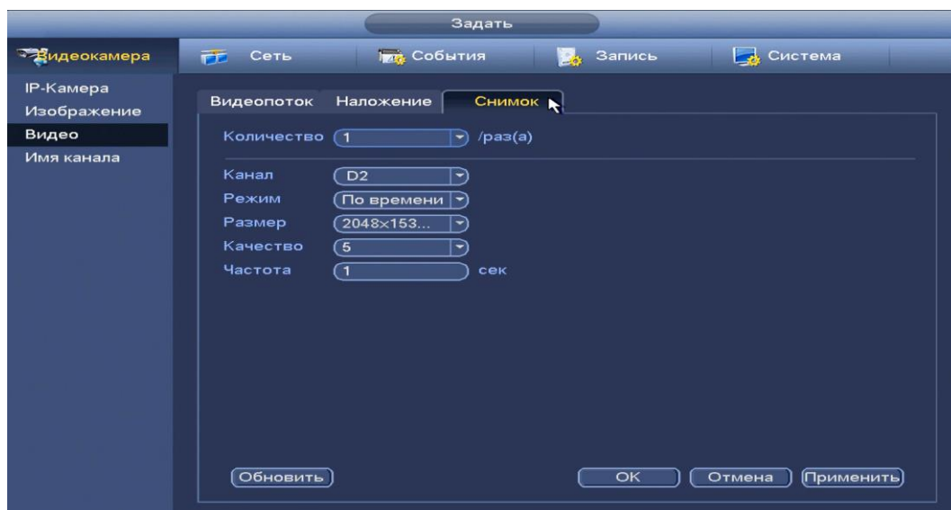
Рисунок 8.40 Настройка снимка.
