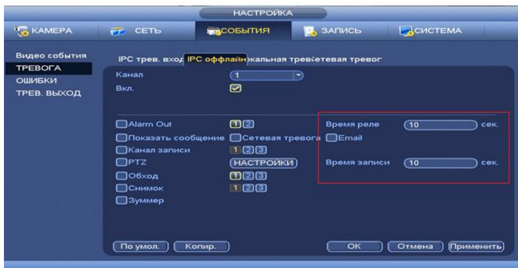
Рисунок 8.87 Установка настроек
