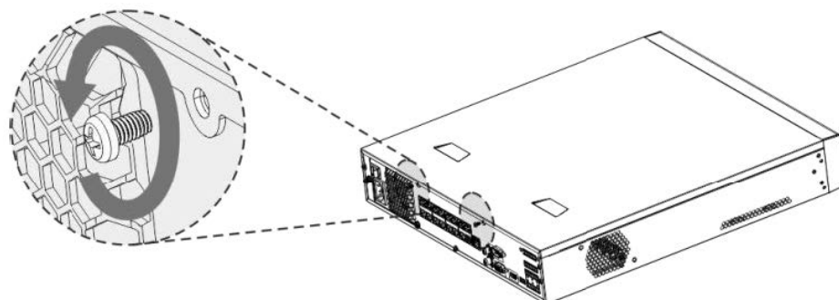
Рисунок 3.3 – Установка жесткого диска
