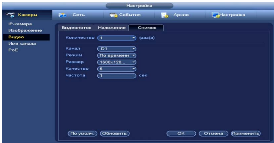
Рисунок 13.5 – Настройка снимка
