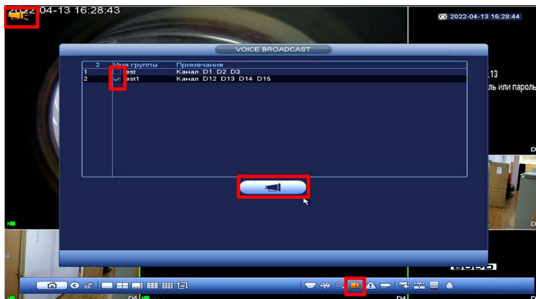
Рисунок 9.4 – Воспроизведение
