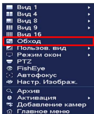
Рисунок 6.2 – Контекстное меню
