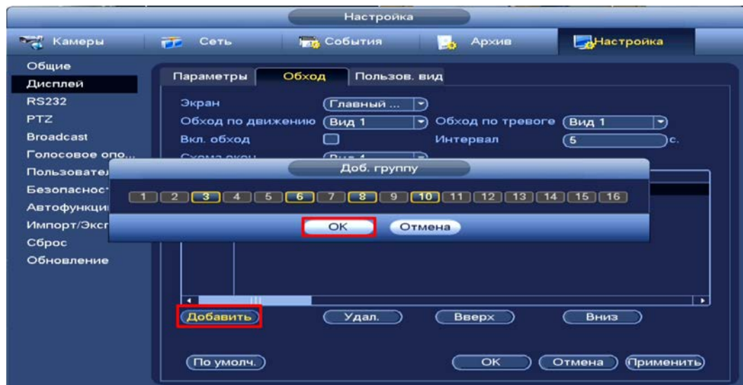
Рисунок 8.7 – Добавление группы
