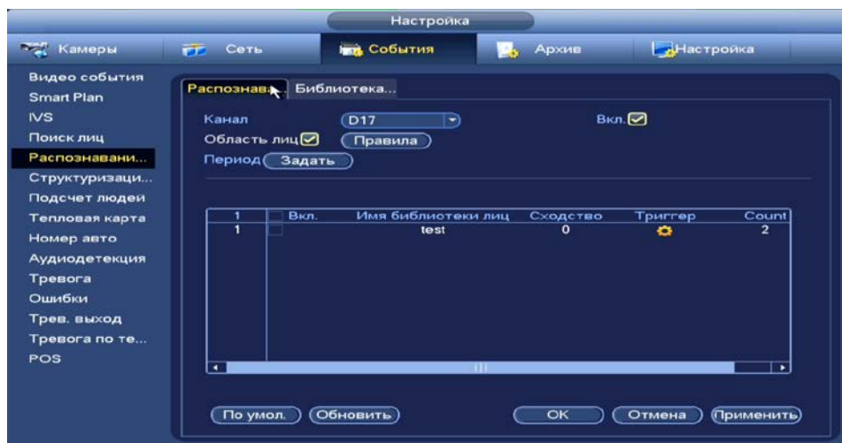
Рисунок 18.17 – Распознавание лиц
