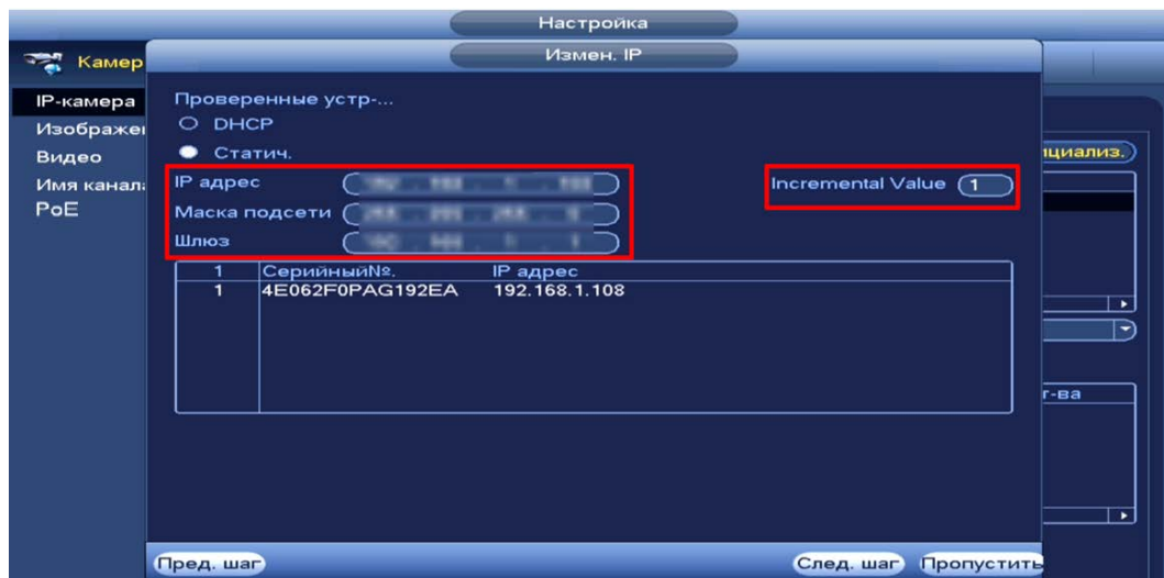
Рисунок 11.8 – Инициализация устройства
