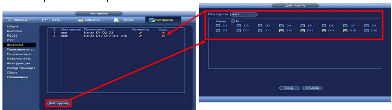
Рисунок 9.3 – Создание группы
