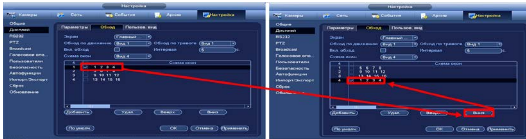
Рисунок 8.6 – Расположение групп
