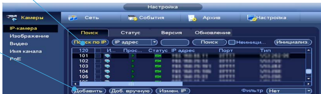
Рисунок 11.4 – Поиск
