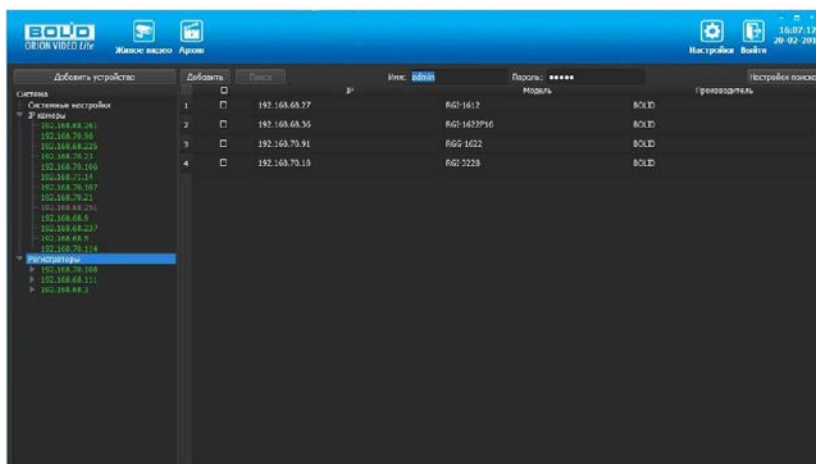
Рисунок 25.4 – Таблица результатов
