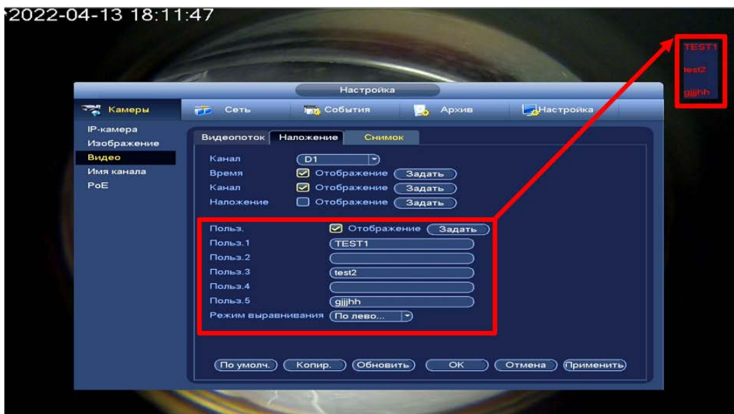
Рисунок 13.7 – Текстовое наложение
