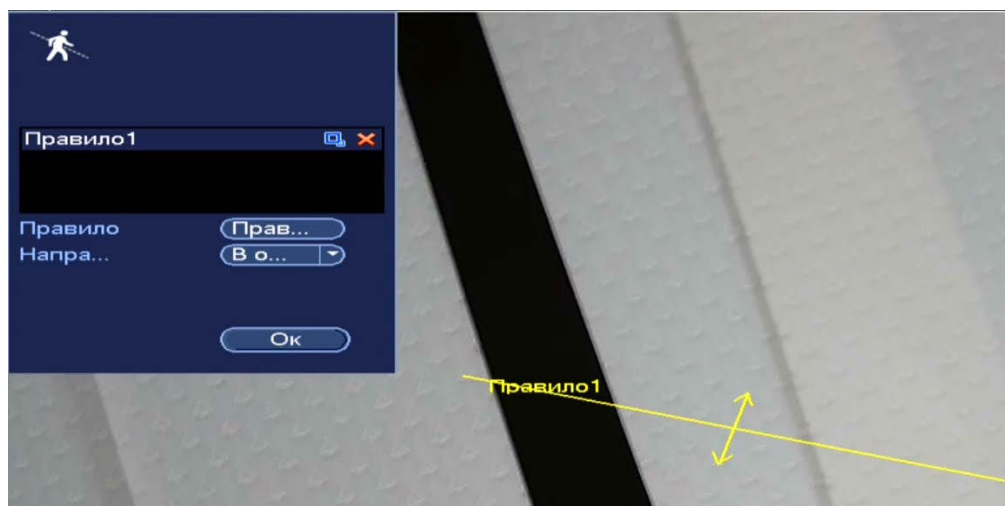
Рисунок 18.3 – Настройка правила
