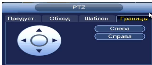
Рисунок 7.7 – Интерфейс «Сканирование»
