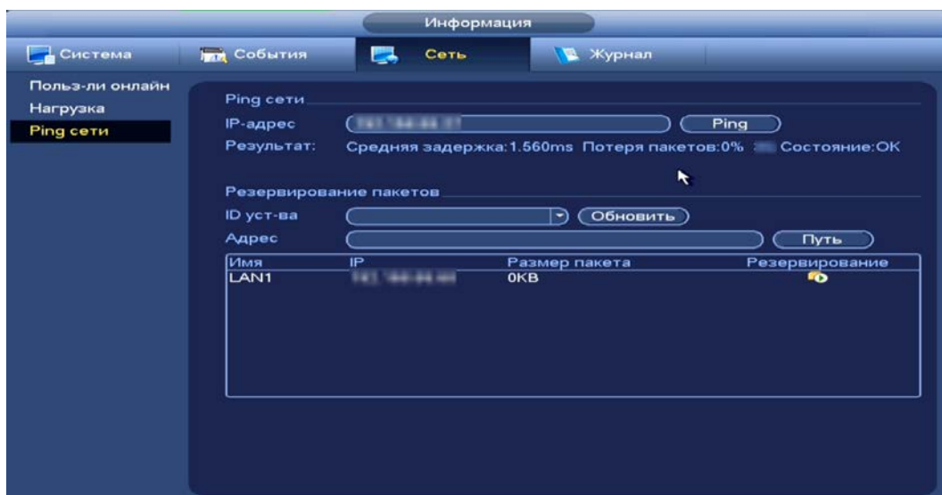
Рисунок 11.18 – Проверка IP-адреса
