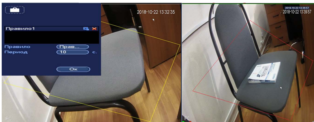
Рисунок 18.9 – Настройка функции
