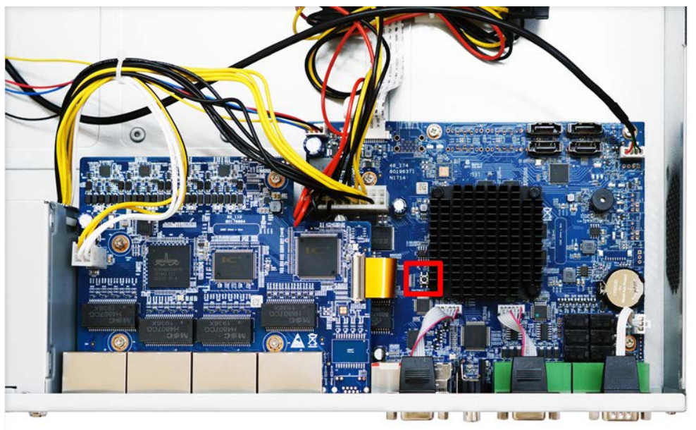
Рисунок 22.10 – Кнопка сброса
