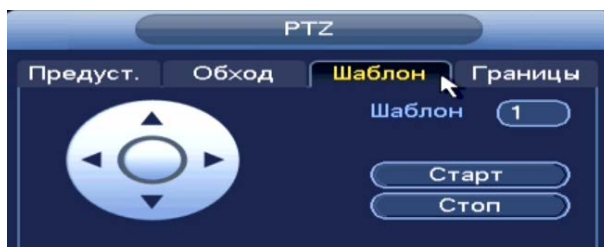
Рисунок 7.6 – Интерфейс «Шаблон»
