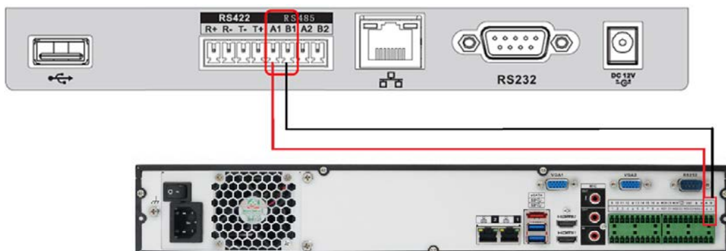
Рисунок 12.4 – Схема RS-485
