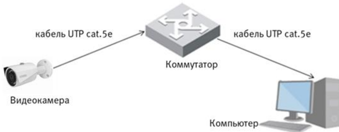
Рисунок 6.3 - Схема подключения видеокамеры к компьютеру через коммутатор
