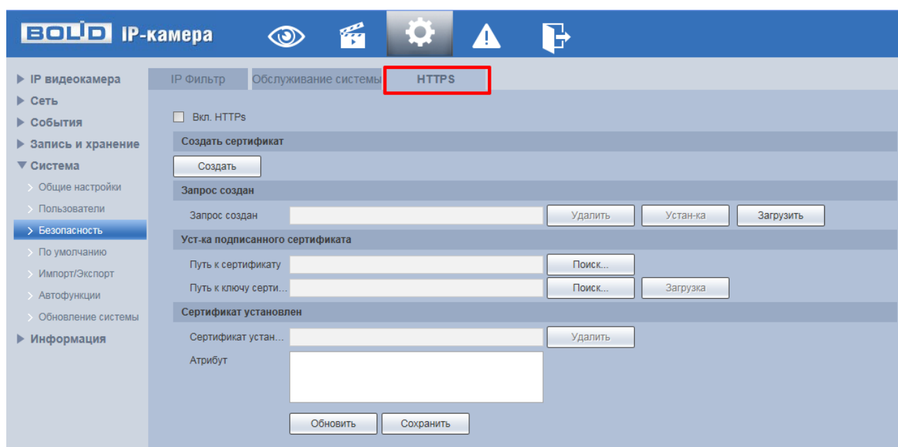
Рисунок 7.112 - Вкладка «HTTPS»
