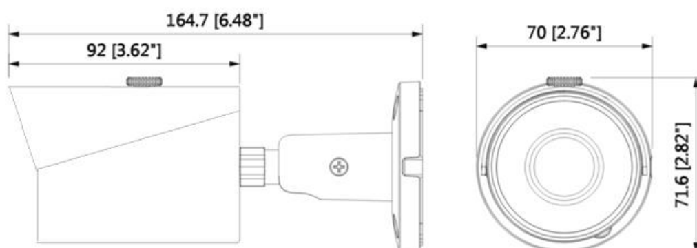
Рисунок 5.1 – Габаритные размеры видеокамеры
