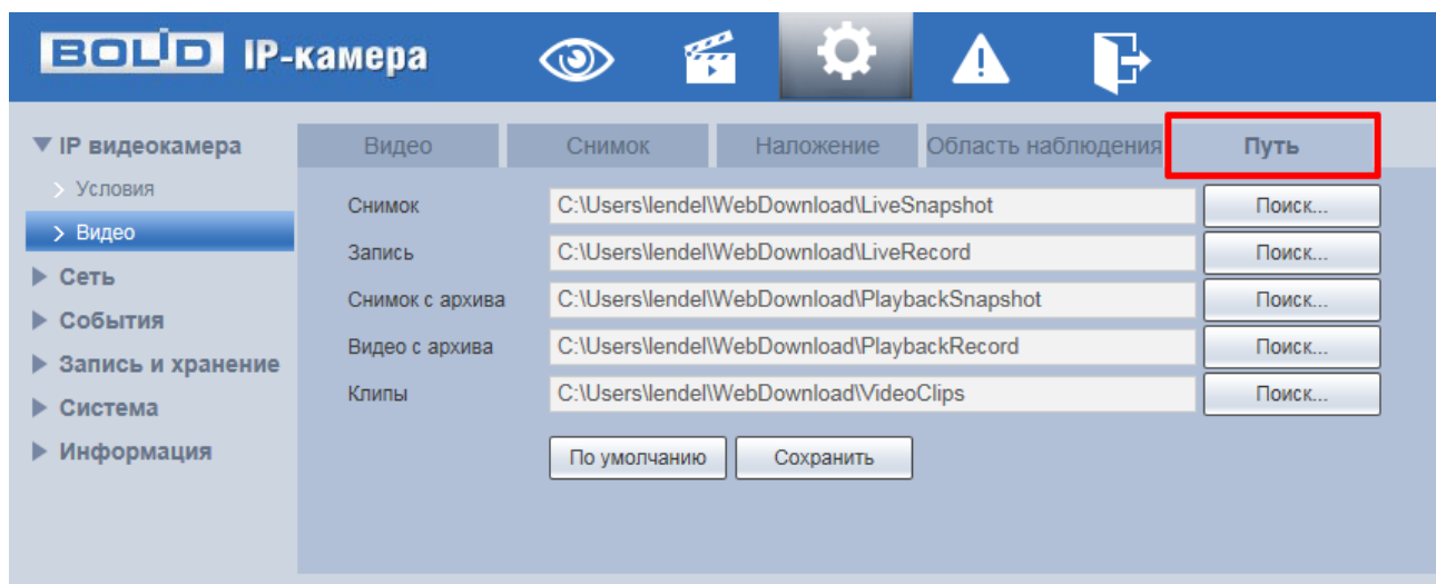
Рисунок 7.48 – Вкладка «Путь»
