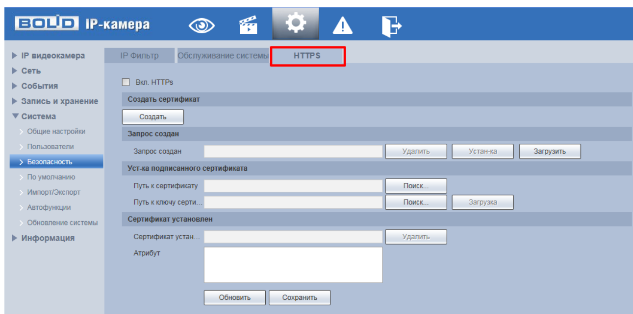
Рисунок 7.111 - Вкладка «HTTPS»
