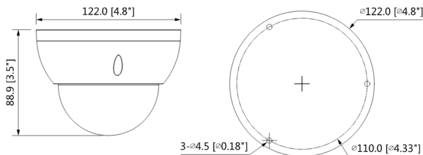
Рисунок 5.1 – Габаритные размеры видеокамеры
