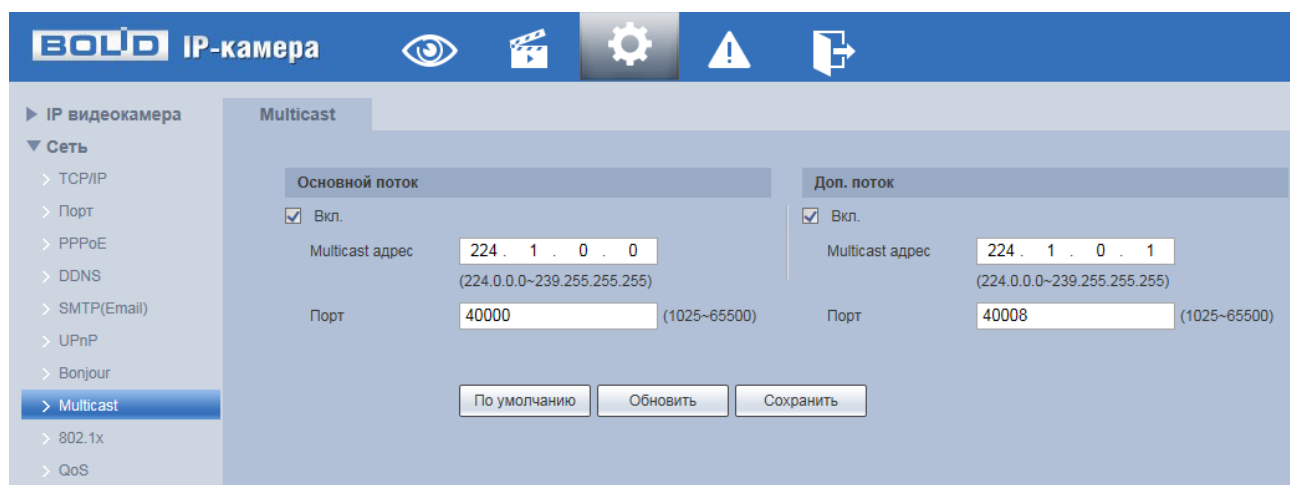
Рисунок 7.63 — Подпункт меню «Multicast»
