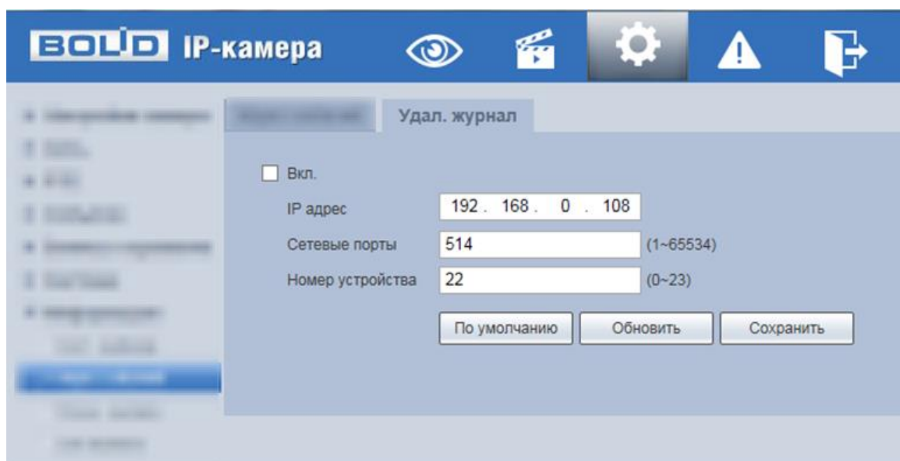
Рисунок 7.128 — Вкладка «Удаленный журнал»
