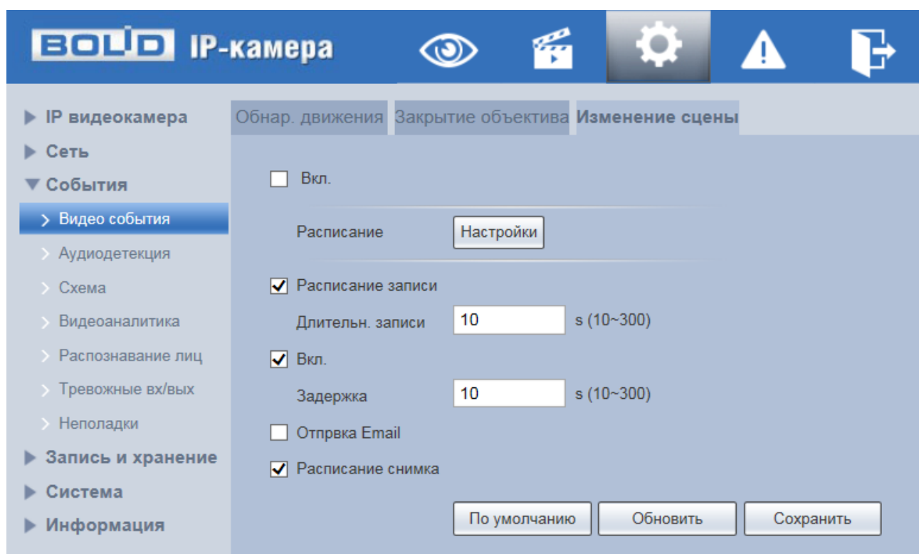
Рисунок 7.78 — Вкладка «Изменение сцены»
