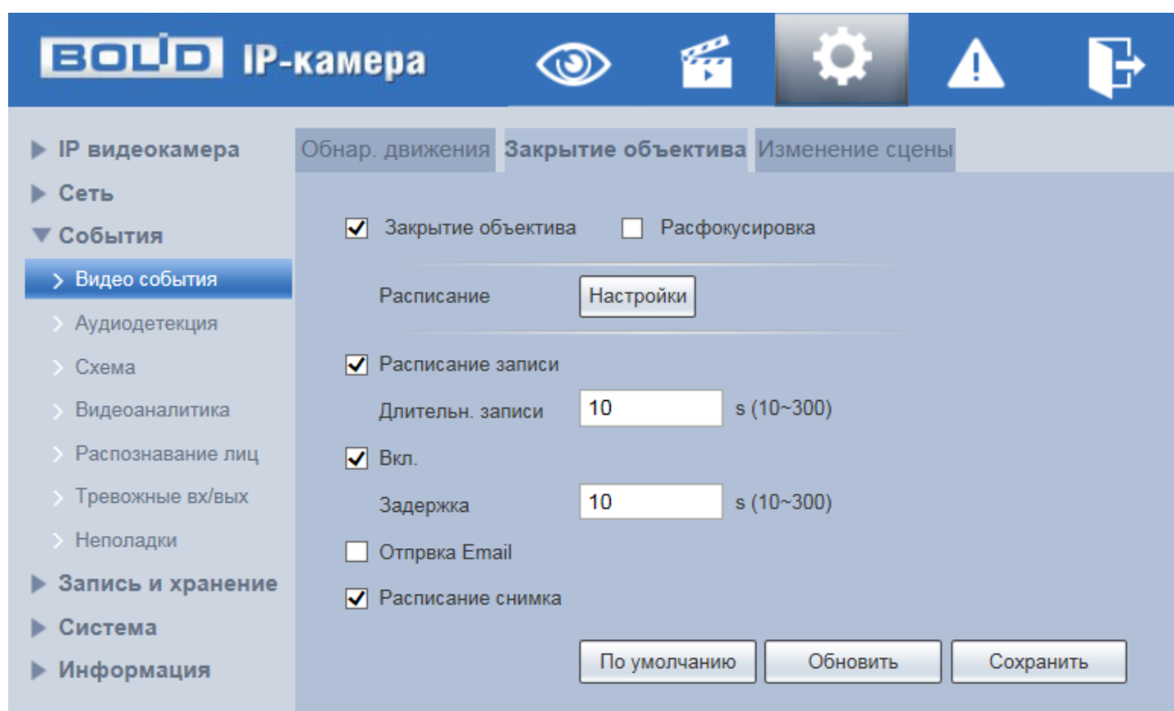
Рисунок 7.76 — Вкладка «Закрытие объектива»
