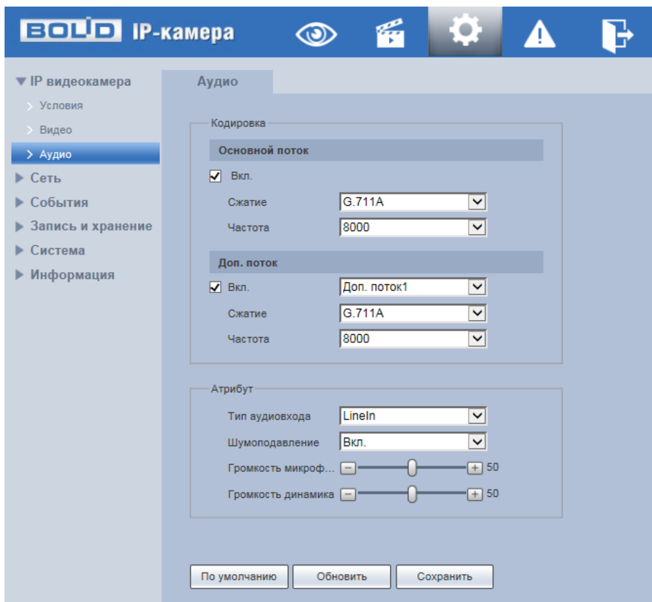
Рисунок 7.50 — Подпункт меню «Аудио»
