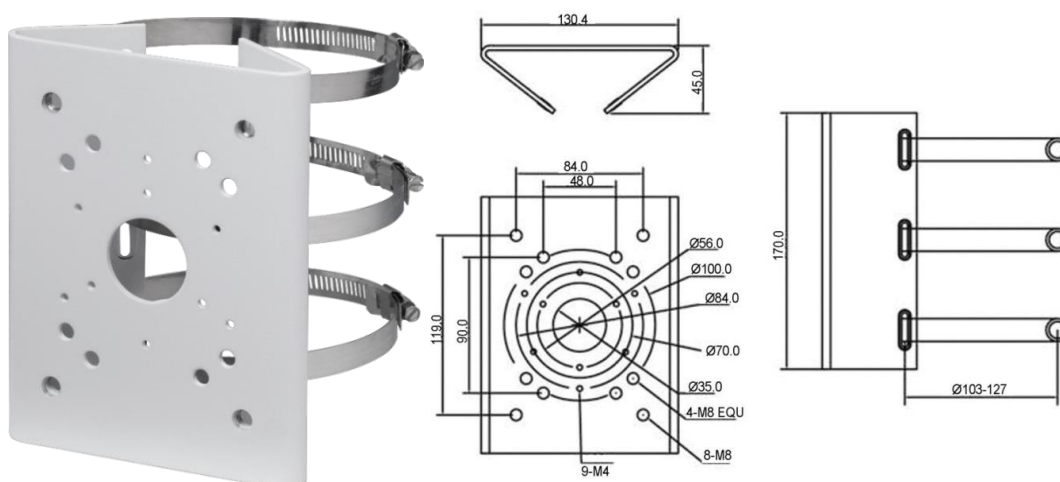
Рисунок 5.13 – Столбовой кронштейн BR-103
