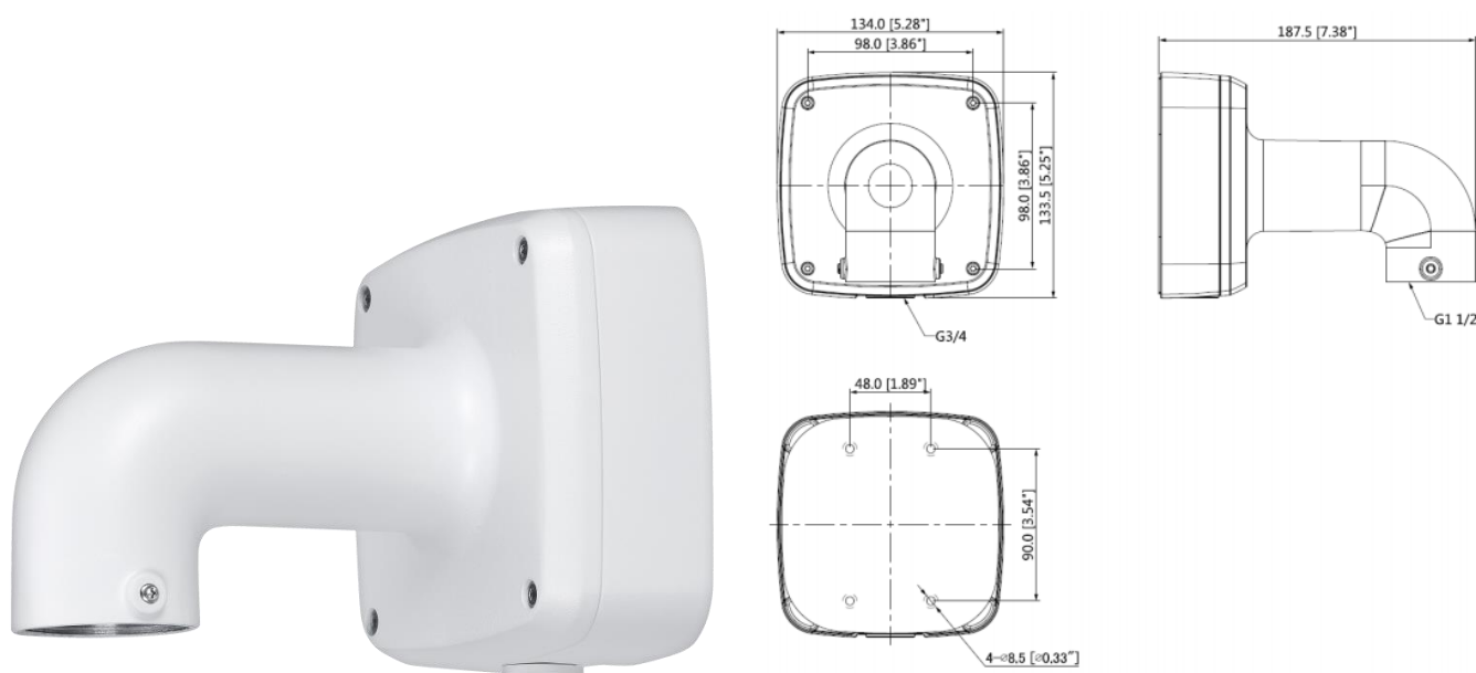
Рисунок 5.8 – Настенный кронштейн BR-107
