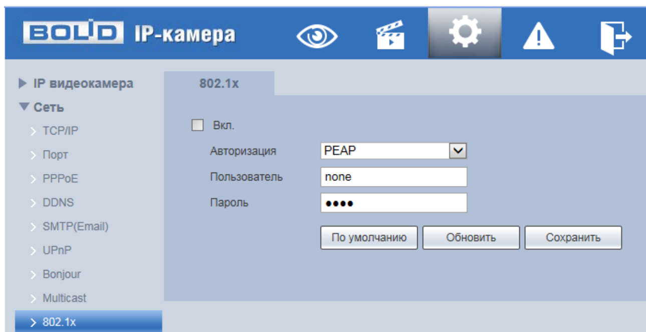
Рисунок 7.64 — Подпункт меню «802.1x»
