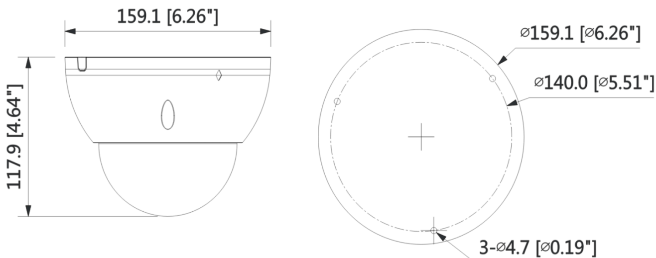
Рисунок 5.1 – Габаритные размеры видеокamеры
