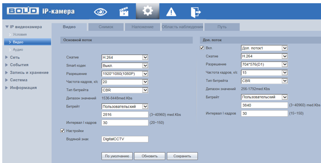
Рисунок 7.39 — Вкладка «Видео»
