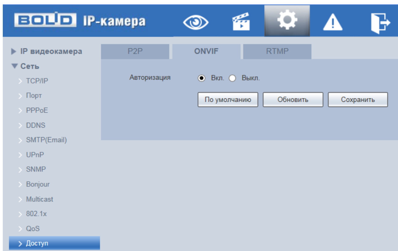
Рисунок 7.68 — Вкладка «ONVIF»
