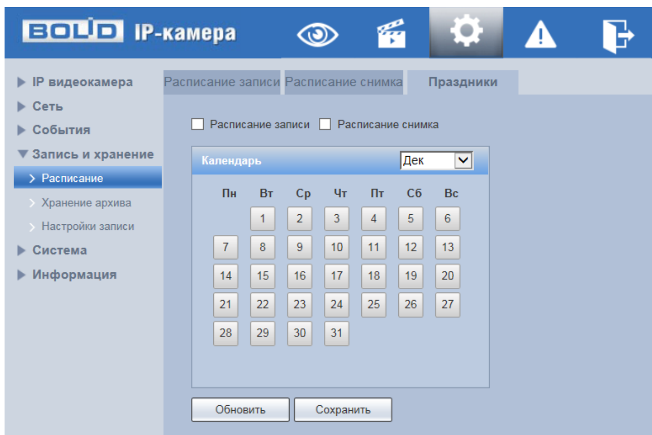
Рисунок 7.98 — Вкладка «Праздники»
