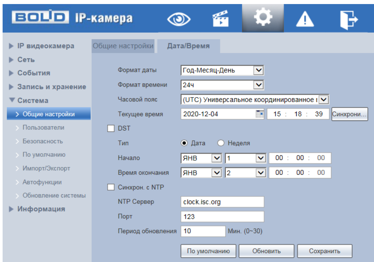
Рисунок 7.109 — Вкладка «Дата/Время»
