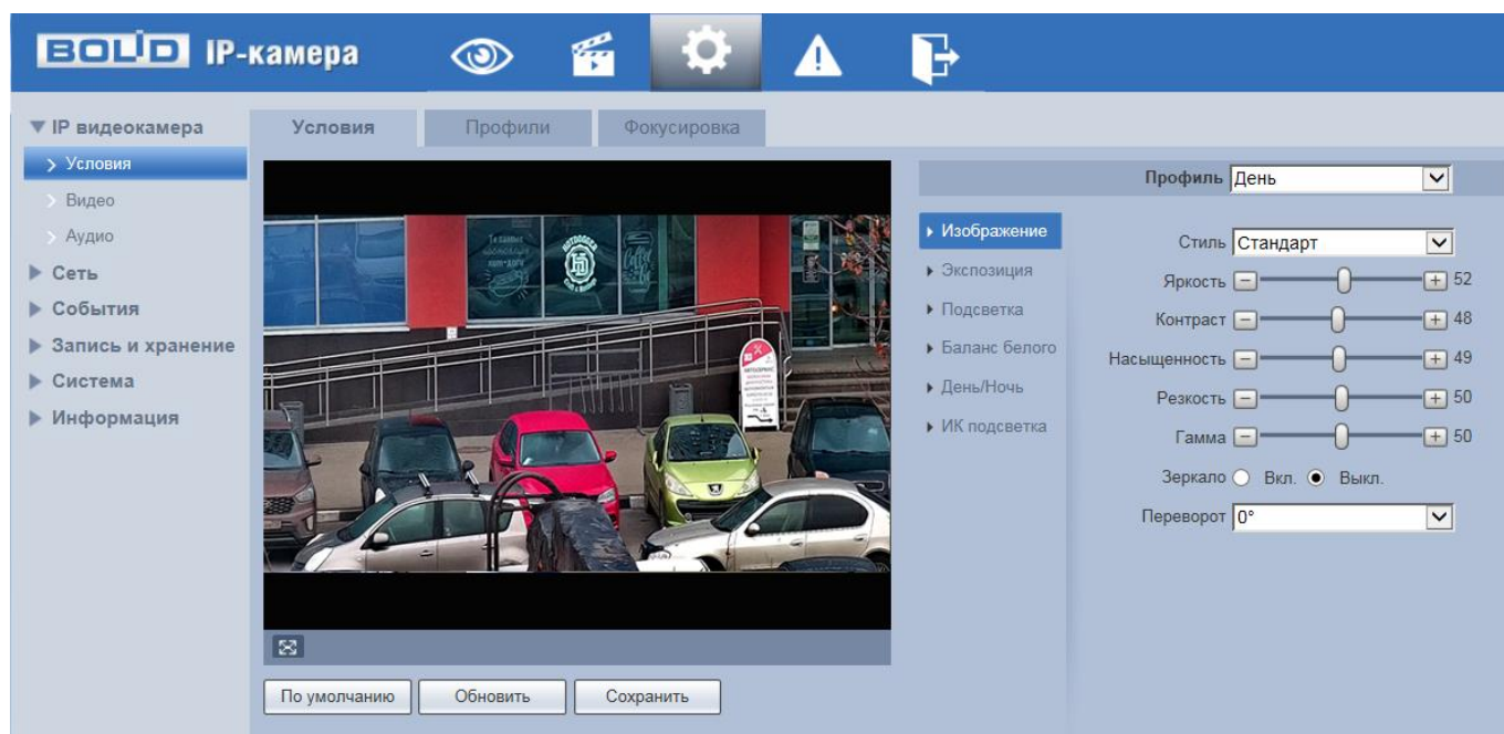
Рисунок 7.27 — Вкладка «Условия»
