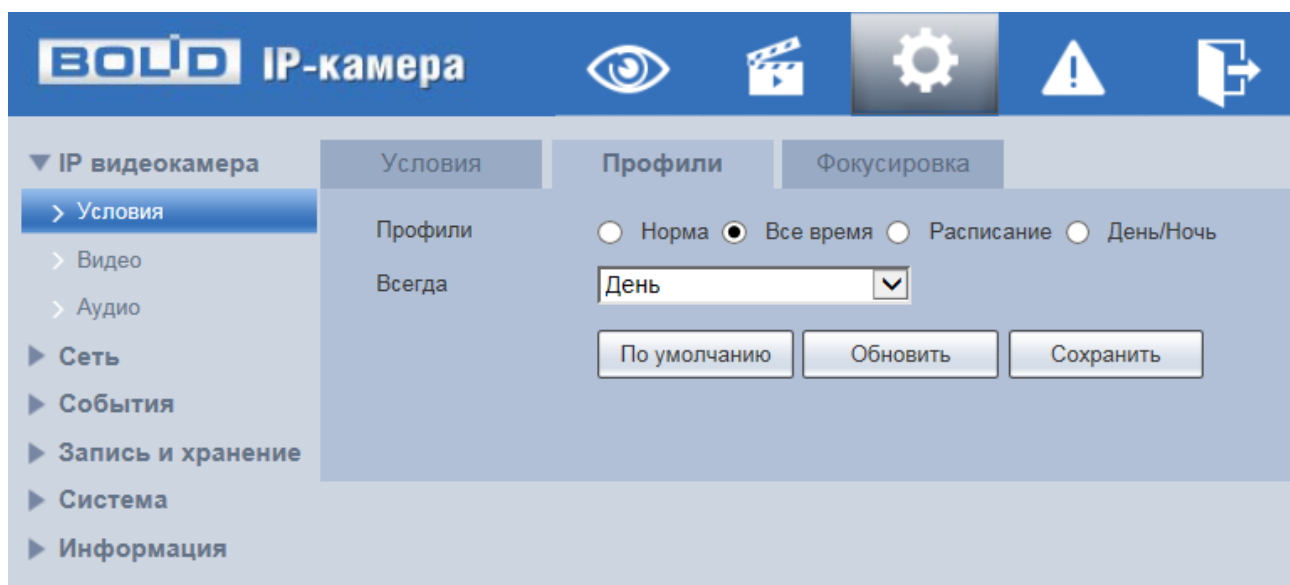
Рисунок 7.36 — Вкладка «Профили»
