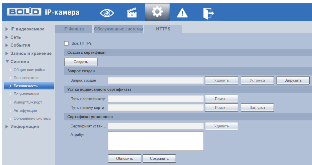
Рисунок 7.117 — Вкладка «HTTPS»
