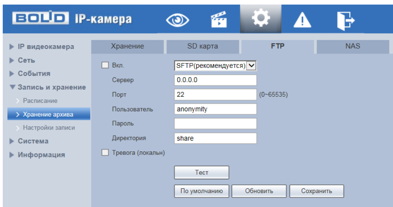
Рисунок 7.102 — Вкладка «FTP»
