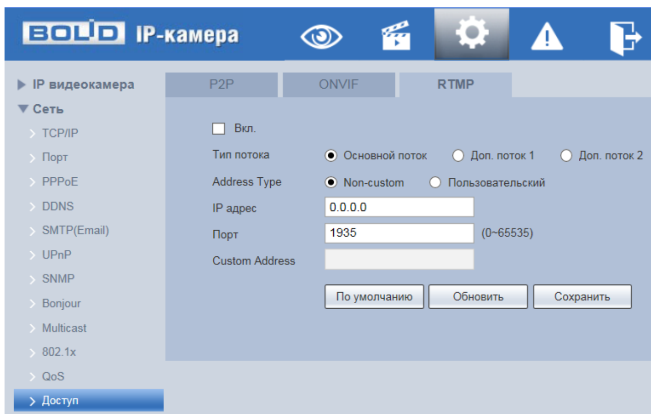
Рисунок 7.69 — Вкладка «RTMP»
