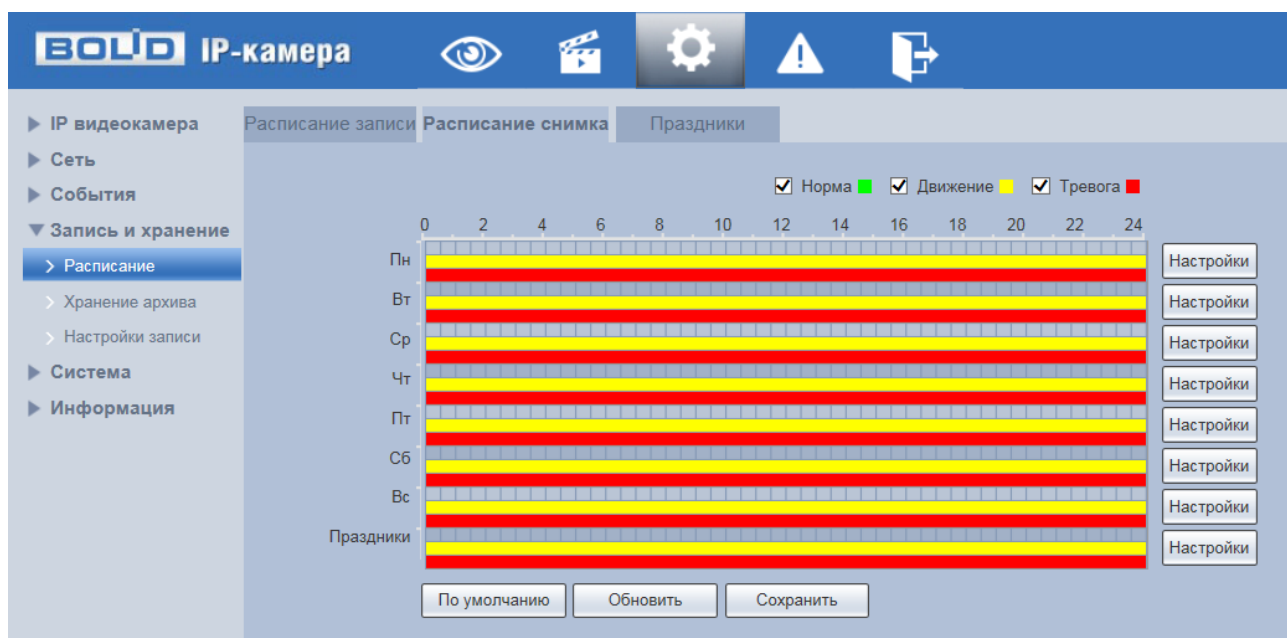
Рисунок 7.96 — Вкладка «Расписание снимка»
