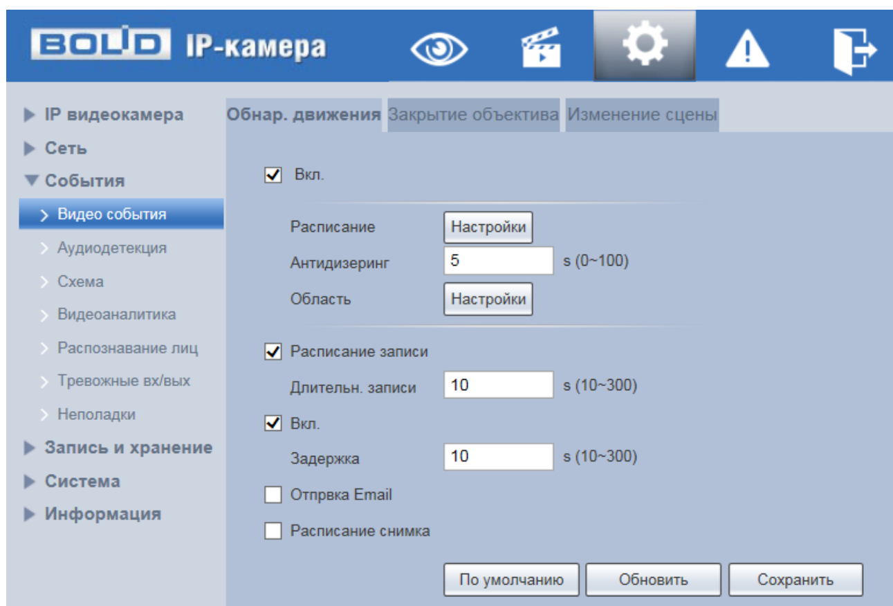
Рисунок 7.73 — Вкладка «Обнаружение движения»
