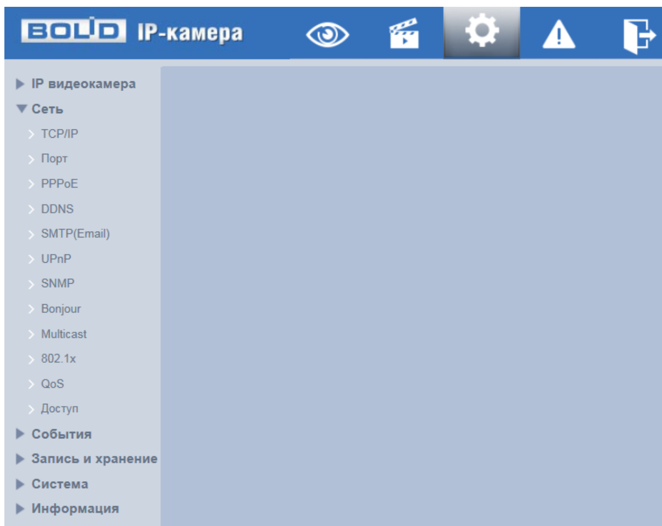
Рисунок 7.51 — Пункт меню «Сеть»
