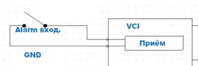
Рисунок 6.6 — Схема подключения тревожного входа
