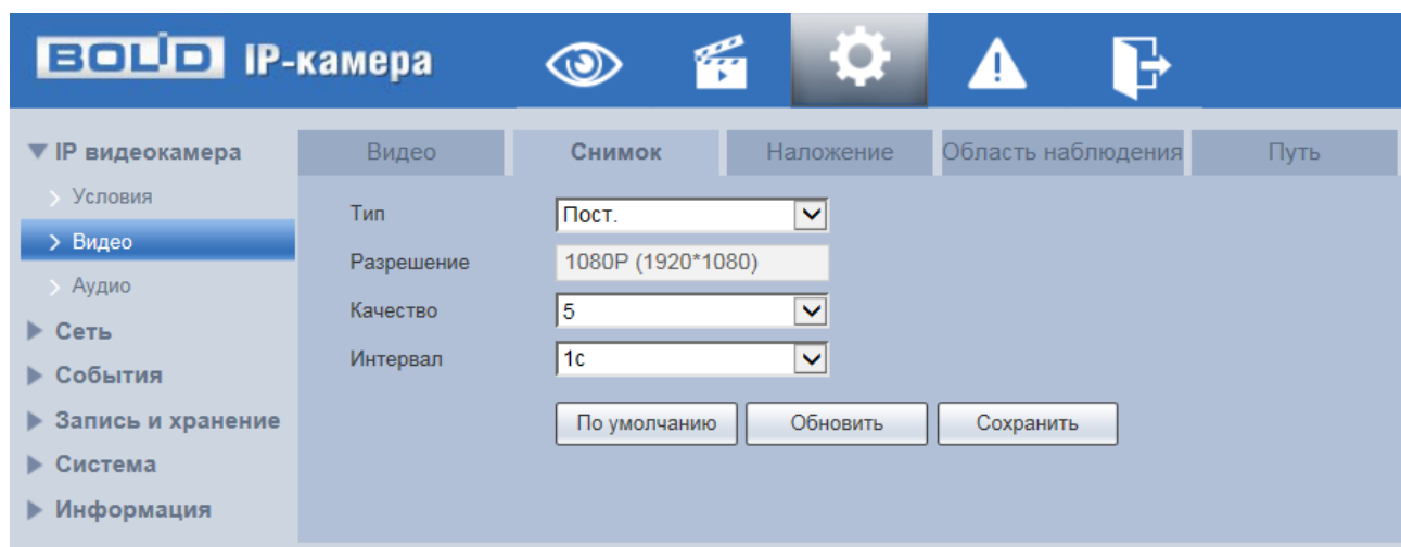
Рисунок 7.40 — Вкладка «Снимок»
