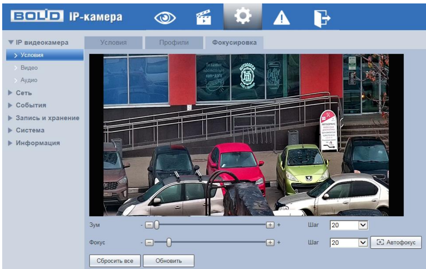
Рисунок 7.37 — Вкладка «Фокусировка»
