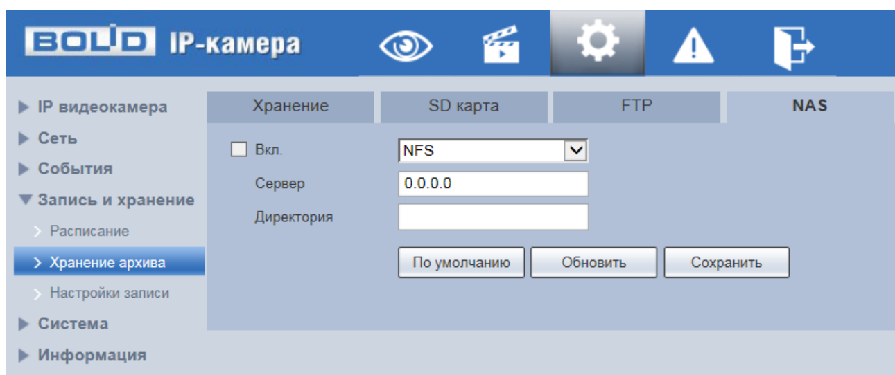
Рисунок 7.103 — Вкладка «NAS»
