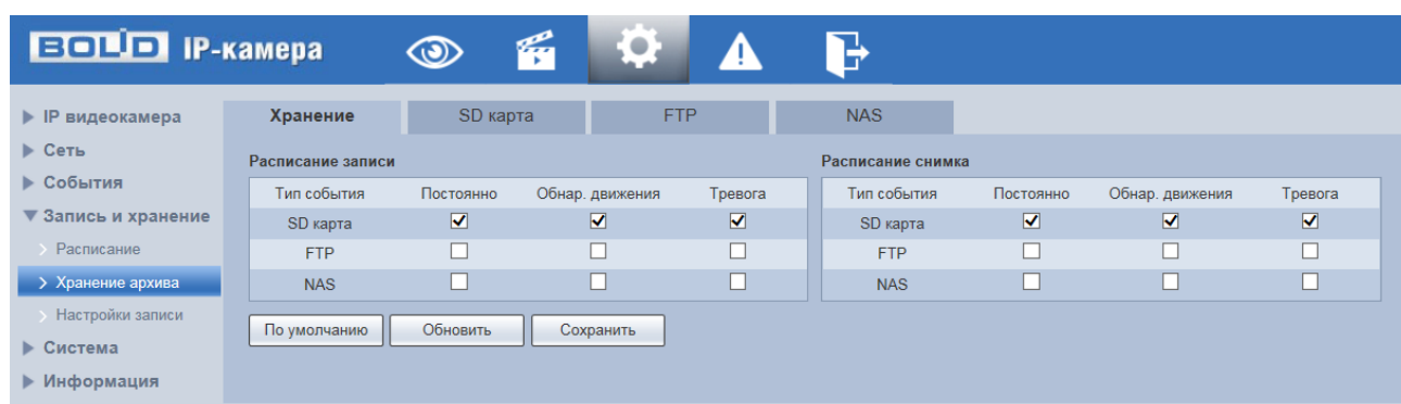
Рисунок 7.100 — Вкладка «Хранение»
