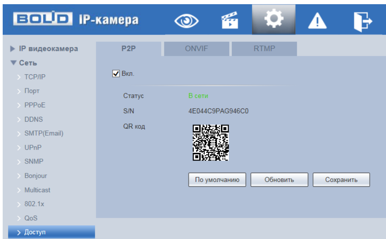
Рисунок 7.67 — Вкладка «P2P»
