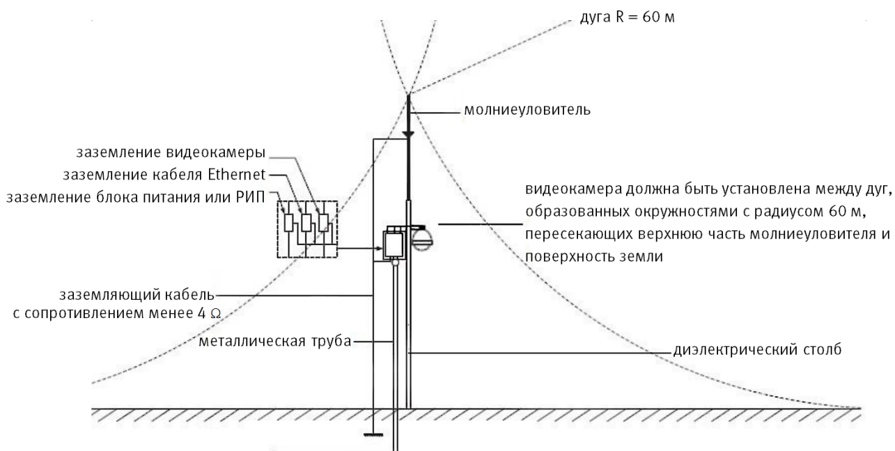
Рисунок 6.7 — Установка молниеотвода
