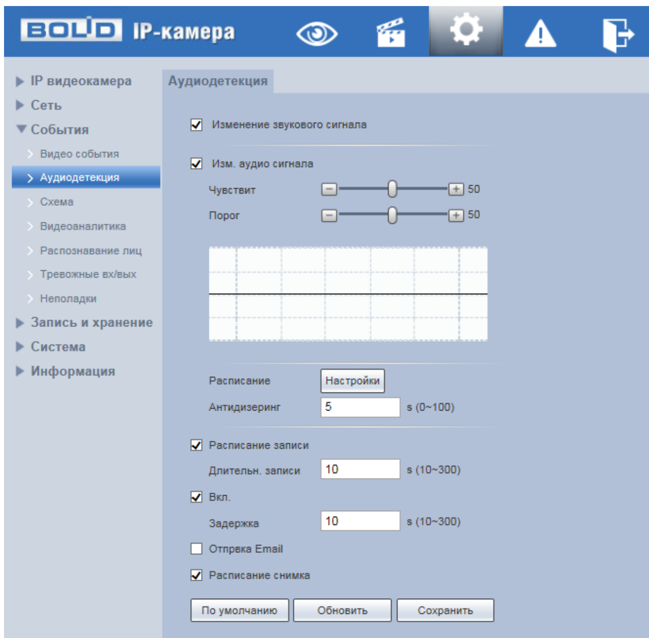
Рисунок 7.80 — Подпункт меню «Аудиодетекция»
