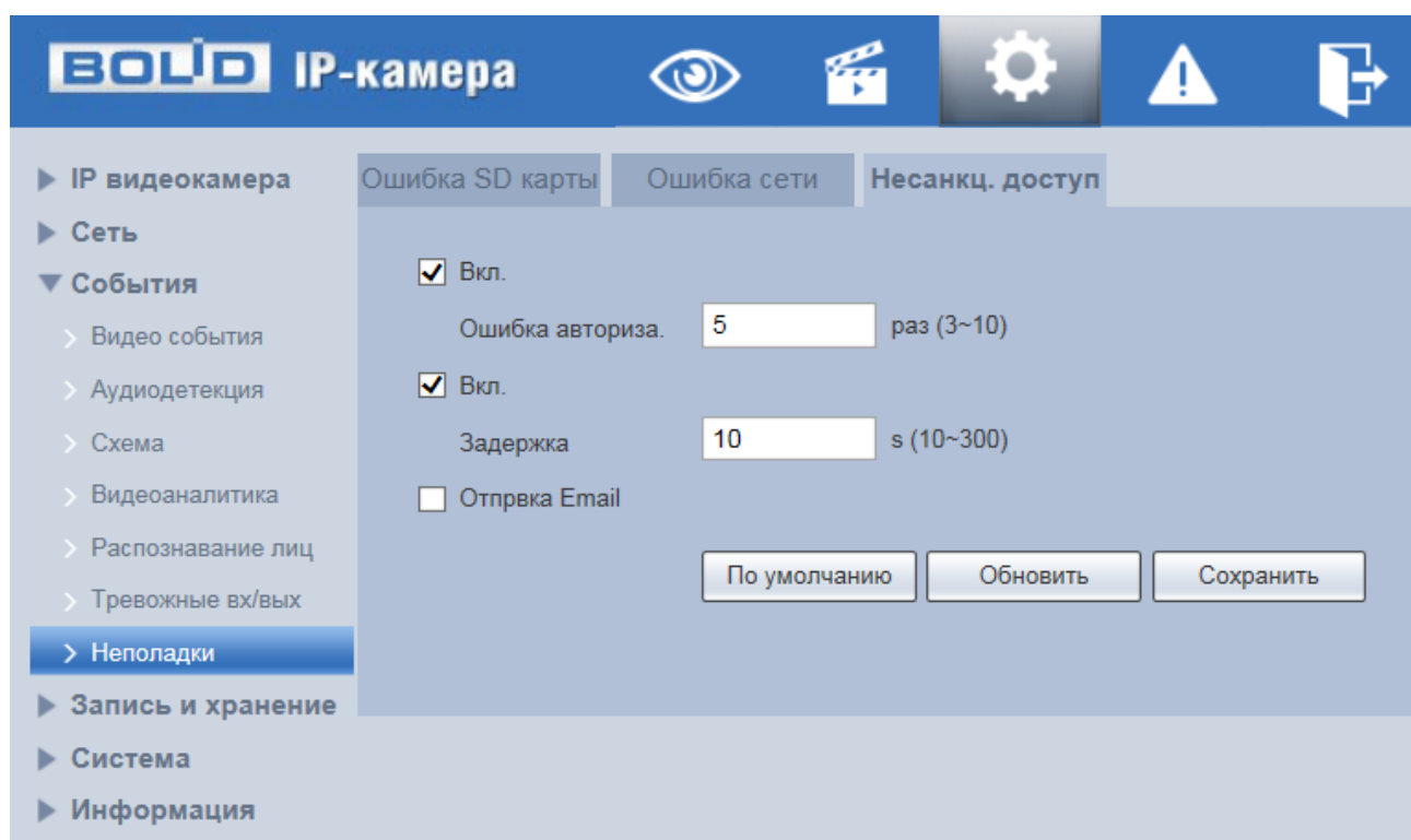
Рисунок 7.90 — Вкладка «Несанкционированный доступ»
