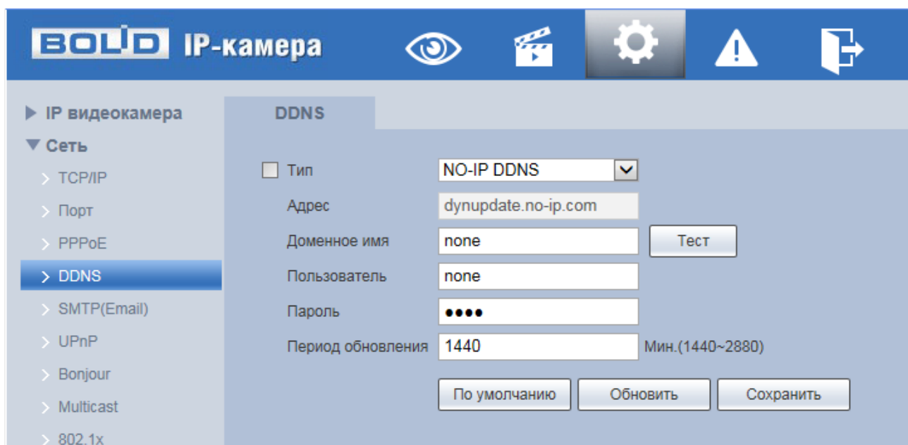
Рисунок 7.56 — Подпункт меню «DDNS»
