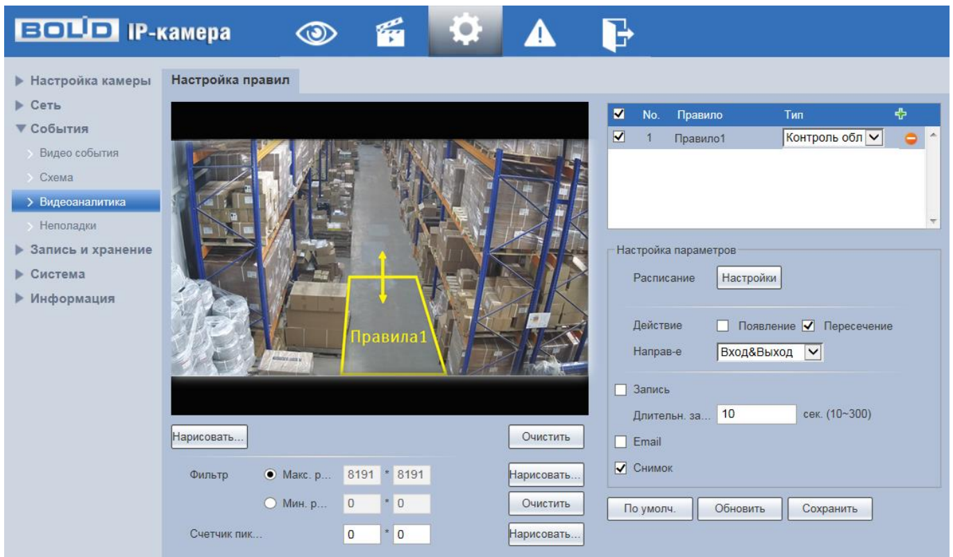
Рисунок 7.84 — Создание правила видеоаналитики «Контроль области»
