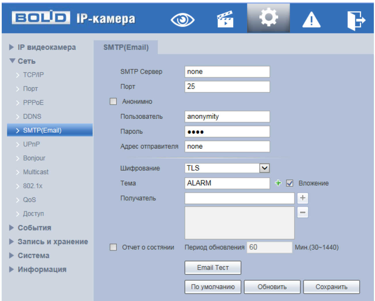
Рисунок 7.58 — Подпункт меню «SMTP»
