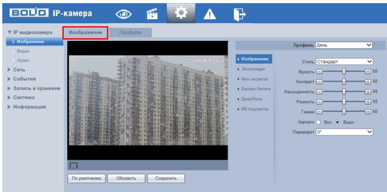
Рисунок 7.22 – Вкладка «Изображение»
