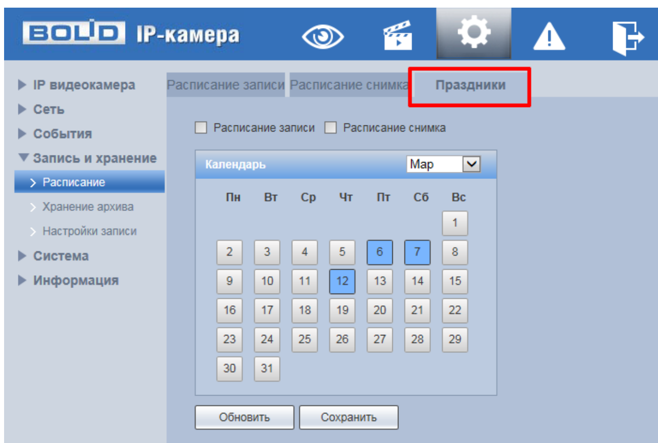
Рисунок 7.88 – Вкладка «Расписание»
