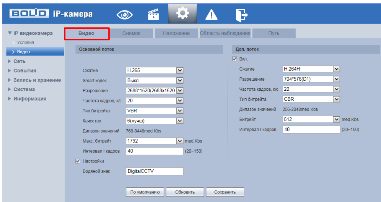
Рисунок 7.32 – Вкладка «Видео»
