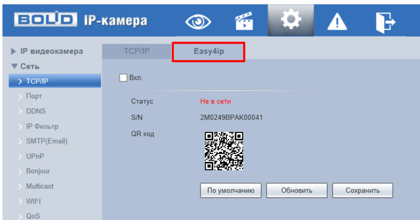
Рисунок 7.47 - Вкладка «Easy4ip»
