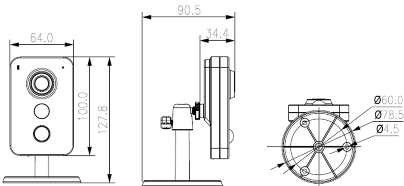
Рисунок 5.1 – Габаритные размеры видеокамеры
