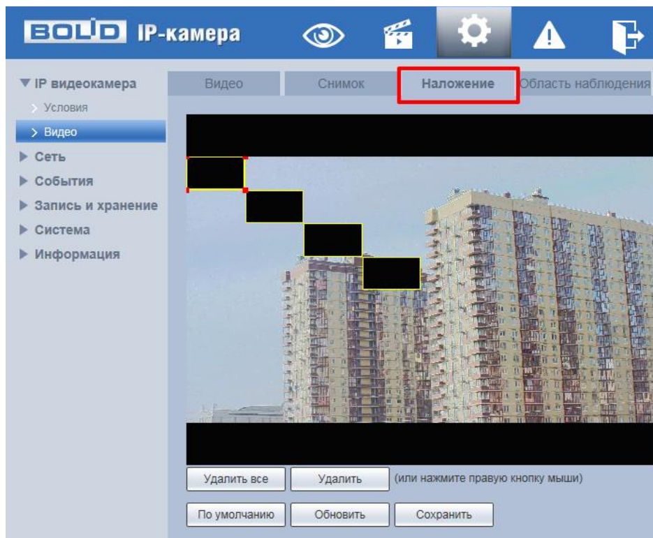
Рисунок 7.34 – Вкладка «Наложение»
