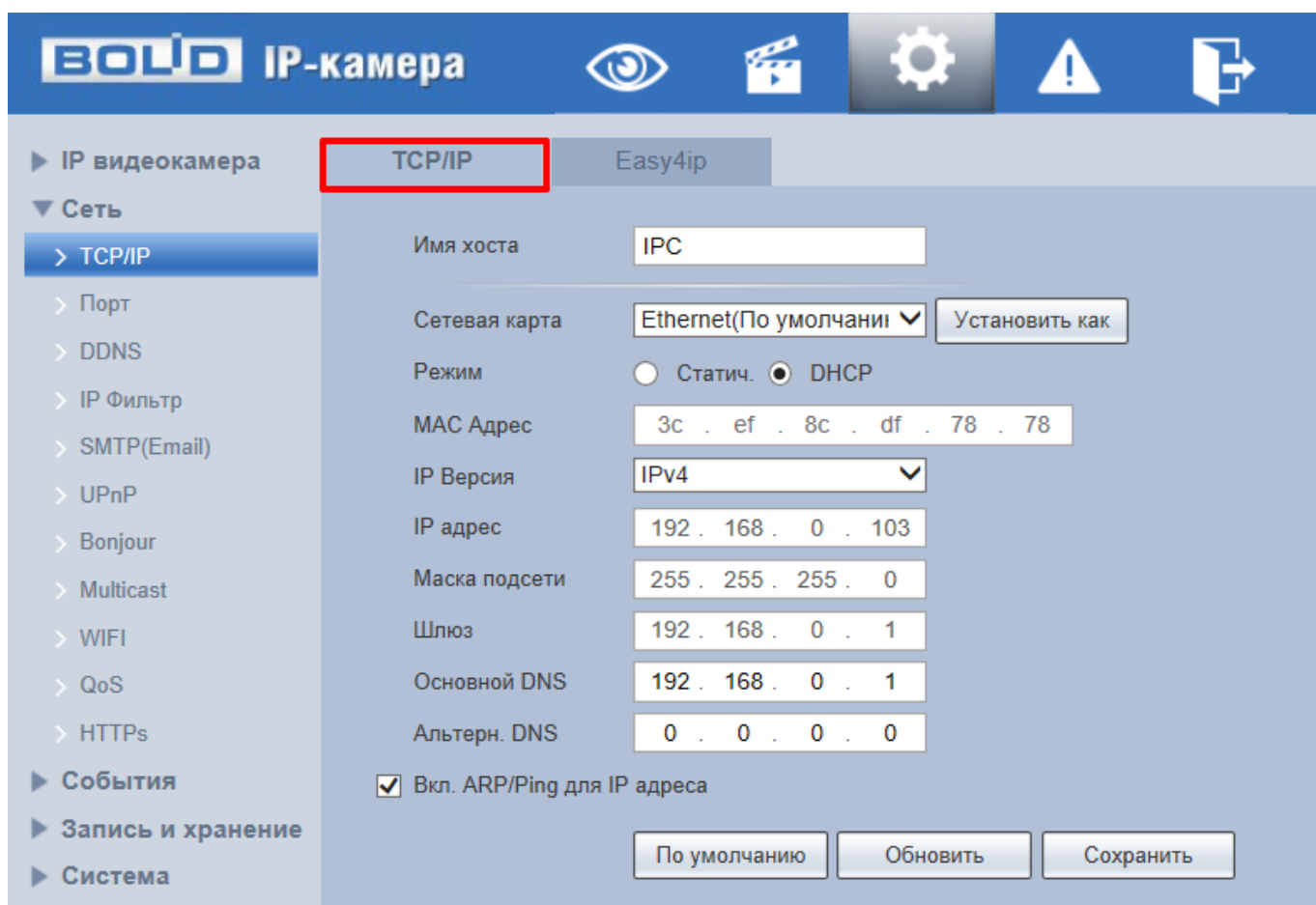
Рисунок 7.46 – Вкладка «TCP/IP»
