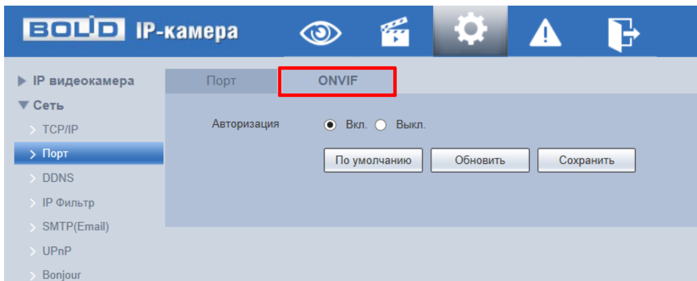
Рисунок 7.49 - Вкладка «ONVIF»
