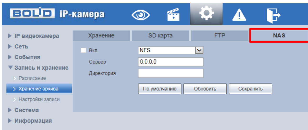
Рисунок 7.93 – Вкладка «NAS»
