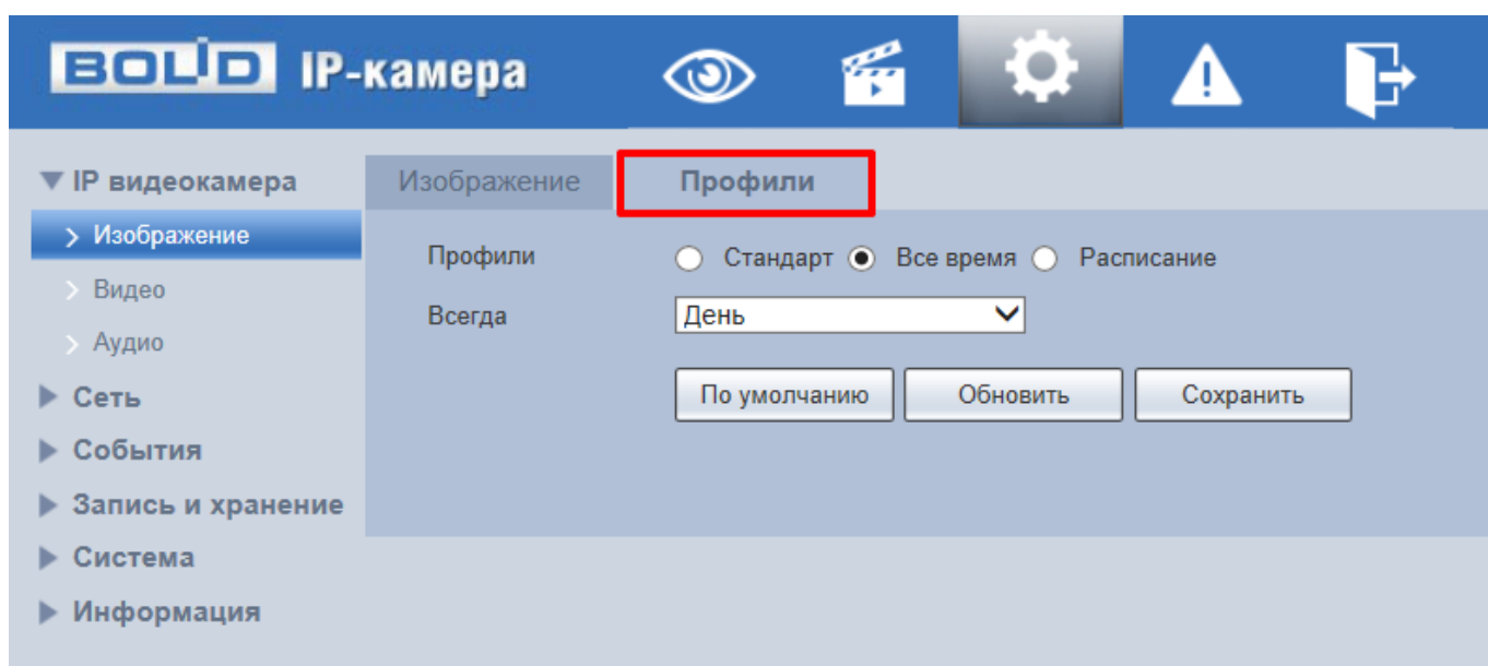
Рисунок 7.30 – Вкладка «Профили»
