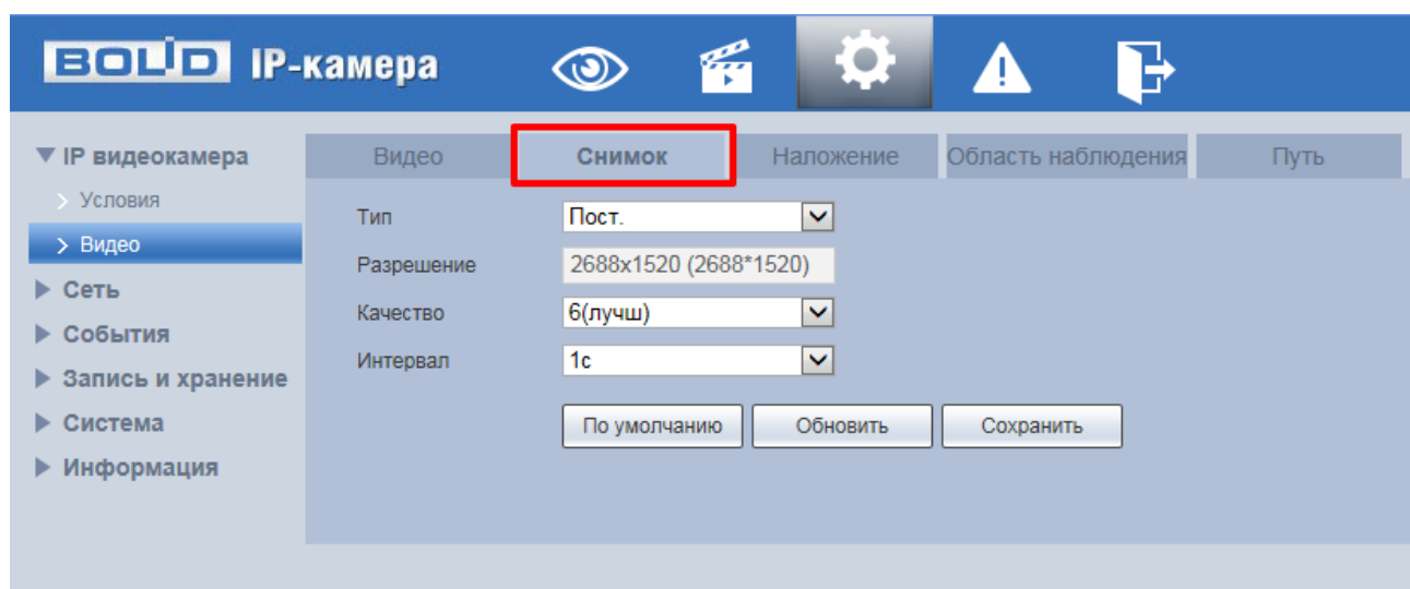
Рисунок 7.33 – Вкладка «Снимок»
