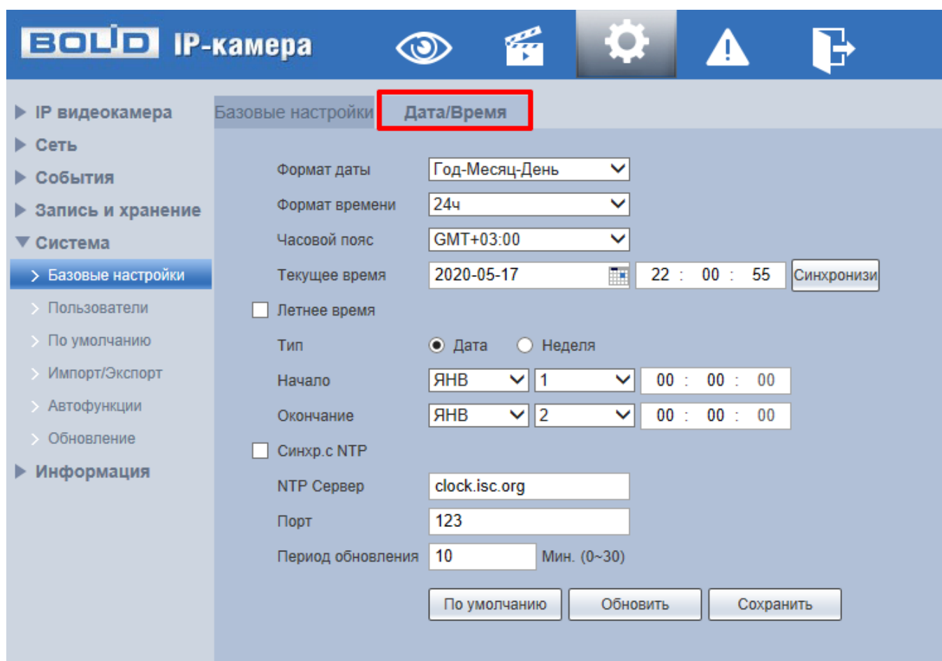
Рисунок 7.99 – Вкладка «Дата/Время»
