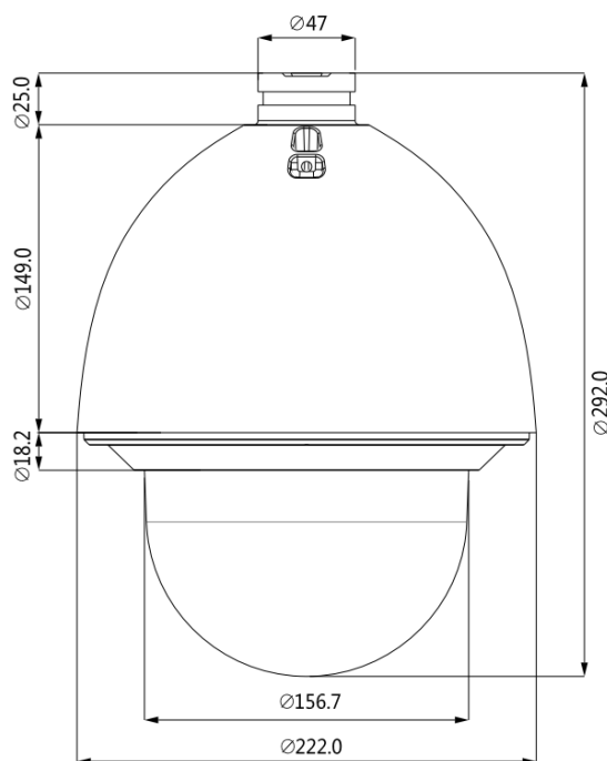
Рисунок 5.1 – Габаритные размеры видеокамеры (мм)
