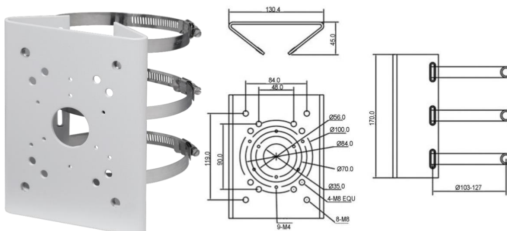
Рисунок 5.15 – Столбовой кронштейн BR-103
