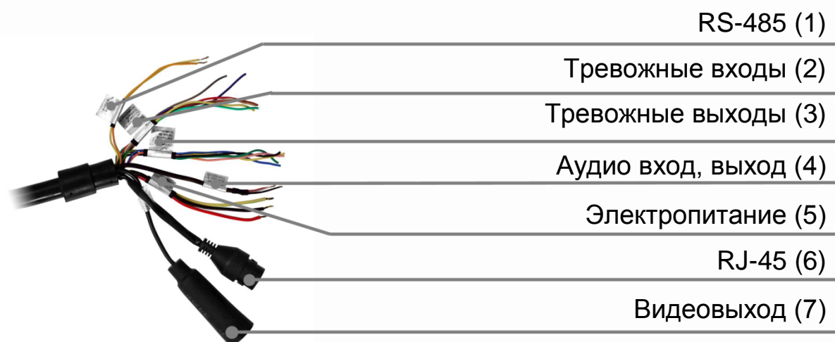
Рисунок 6.1 – Группы концевой раскладки кабеля видеокamеры
