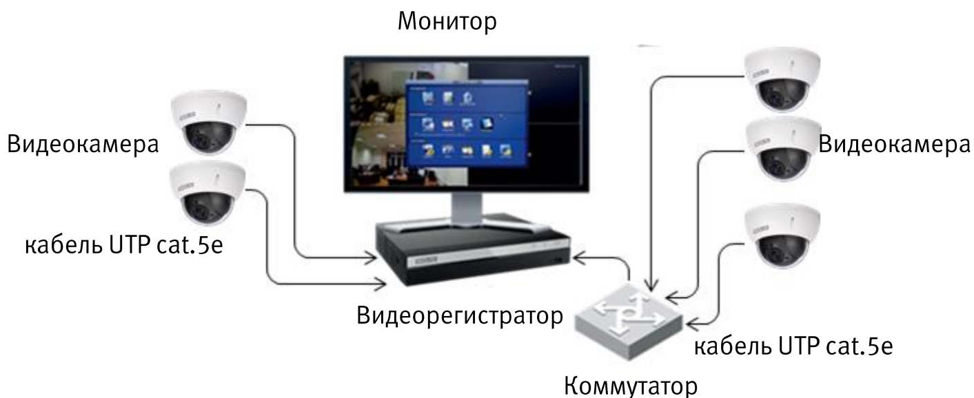
Рисунок 6.4 – Схема подключения видеокамеры к видеорегистратору
