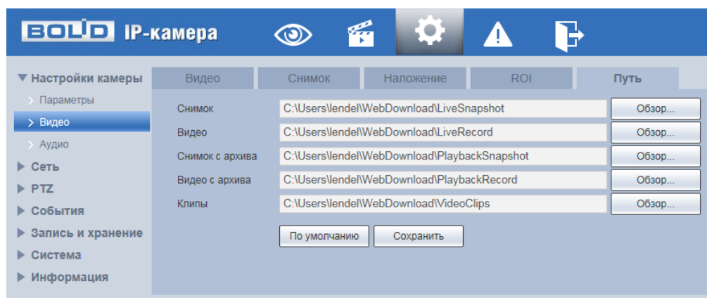
Рисунок 7.49 – Вкладка «Путь»
