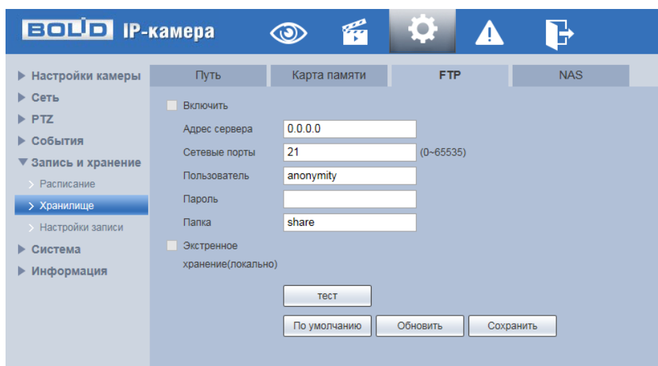
Рисунок 7.140 – Вкладка «FTP»
