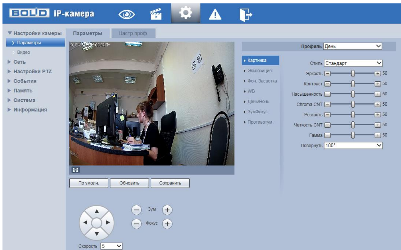
Рисунок 7.25 – Вкладка «Параметры»
