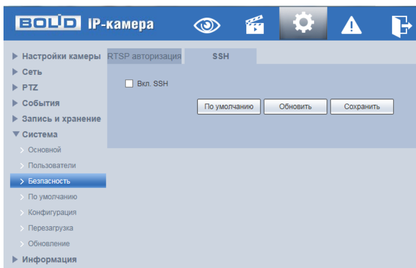
Рисунок 7.154 – Вкладка «SSH»
