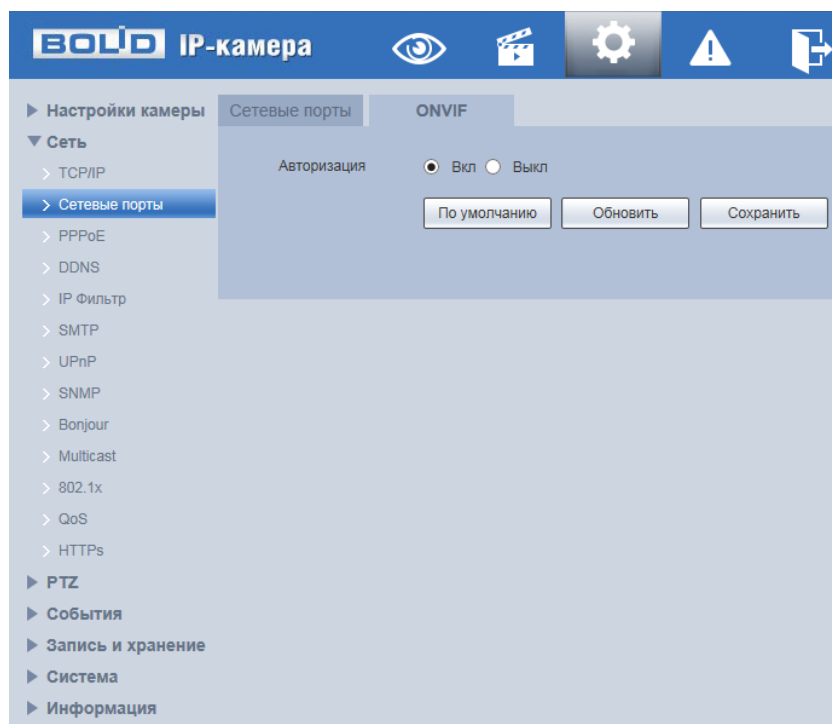
Рисунок 7.55 – Вкладка «ONVIF»
