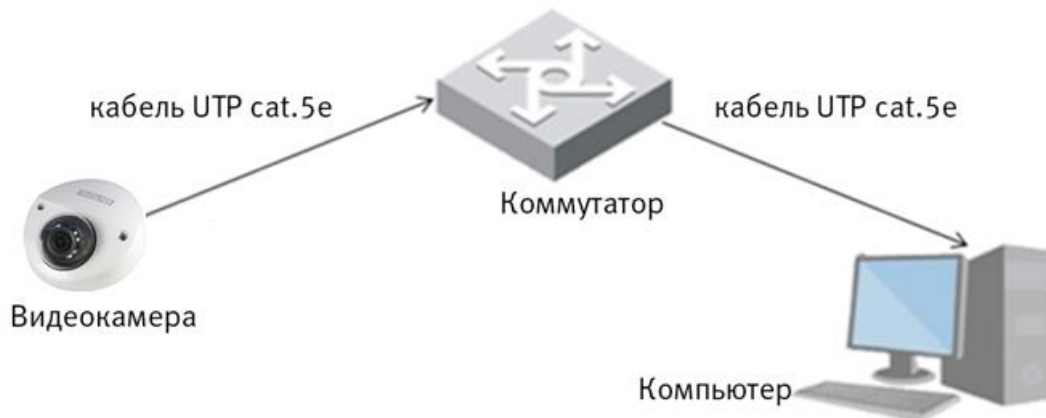
Рисунок 6.3 - Схема подключения видеокамеры к компьютеру через коммутатор
