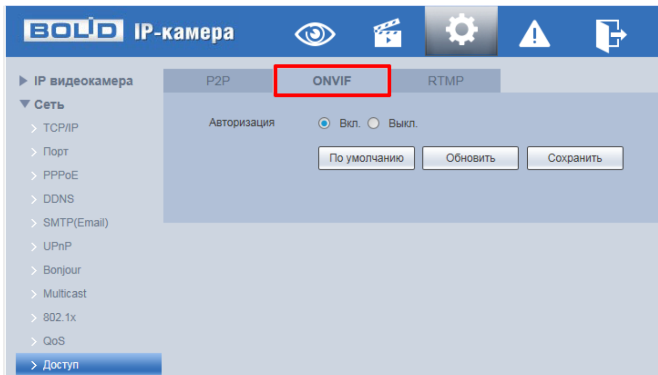
Рисунок 7.65 - Вкладка «ONVIF»
