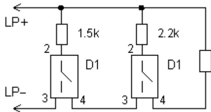
D1: A smoke fire detector
