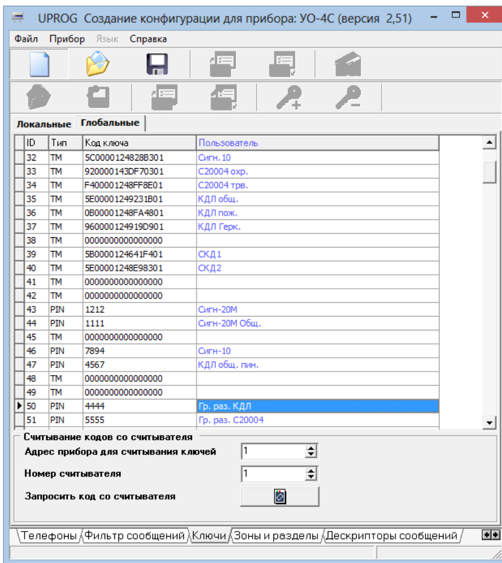
Рисунок 16. Глобальные ключи, мастер режим
