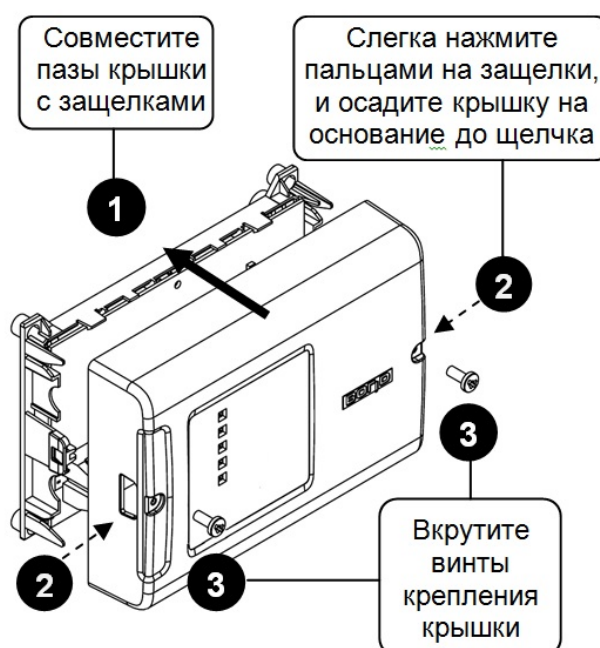
Рисунок 6. Монтаж крышки
