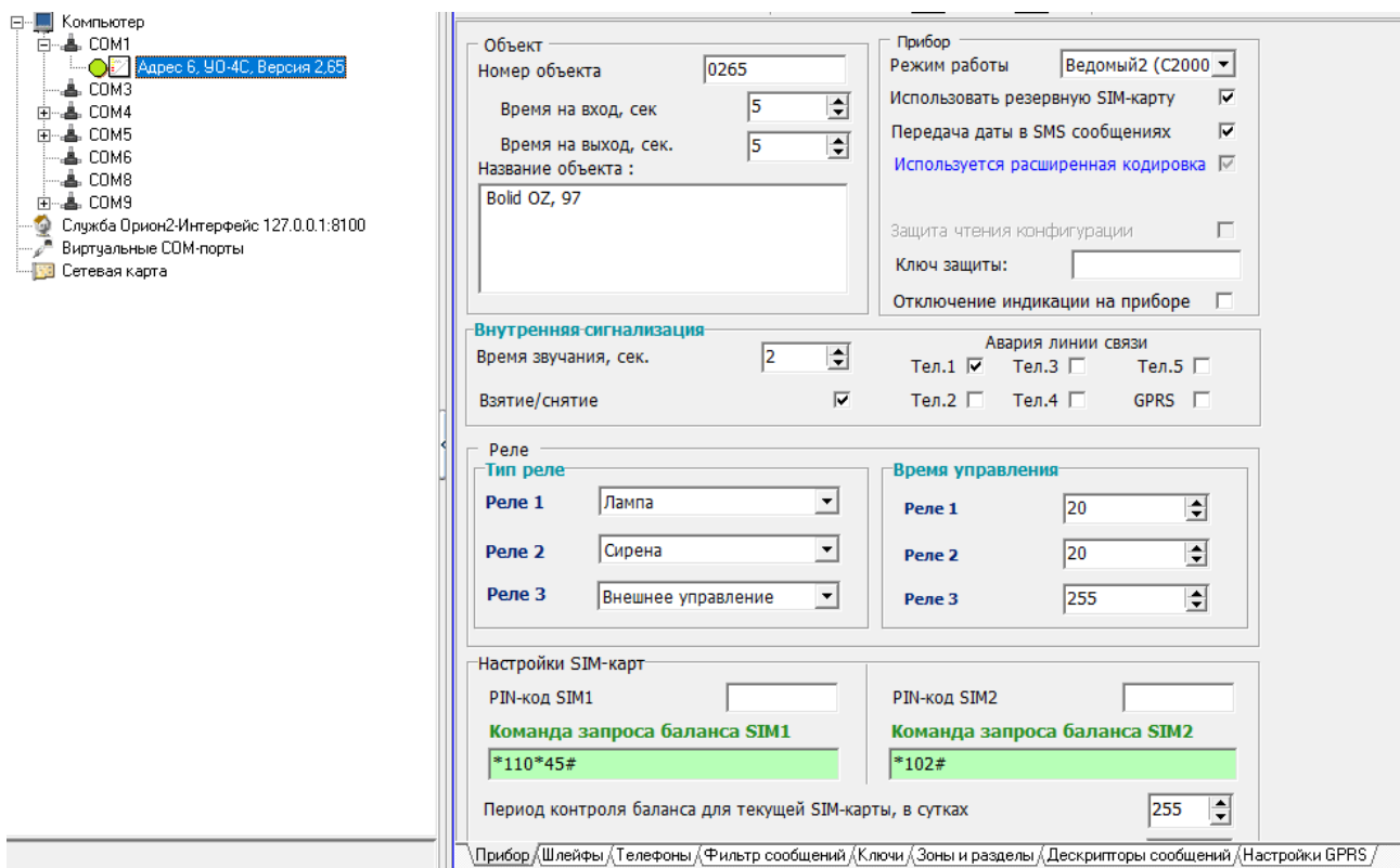
Рисунок 10. Uprog «УО-4С»
