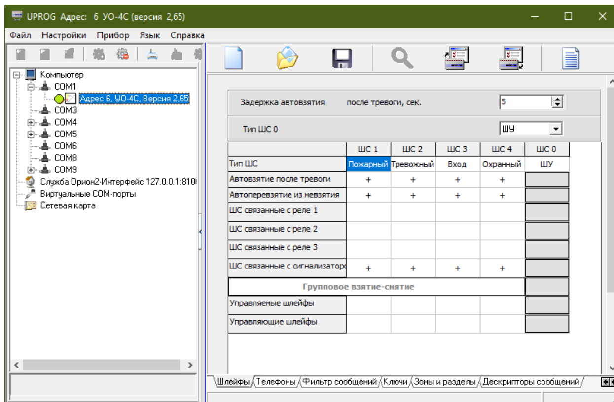
Рисунок 12. «Шлейфы»
