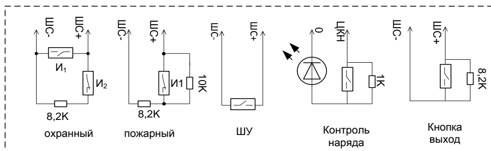
Рисунок 4. Подключение ШС, ШУ
