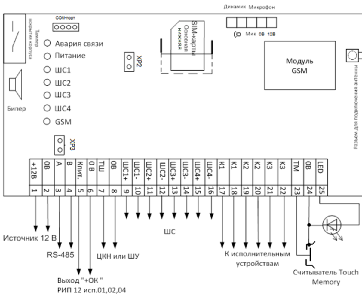
Рисунок 3. Схема подключений прибора «УО-4С»
