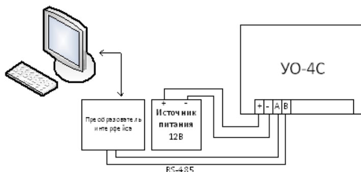
Рисунок 8. Подключение «УО-4С» к ПК через преобразователь интерфейса
