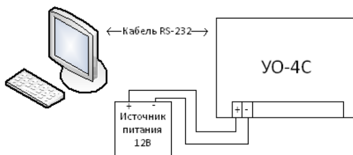
Рисунок 7. Подключение «УО-4С» к ПК через кабель сопряжения
