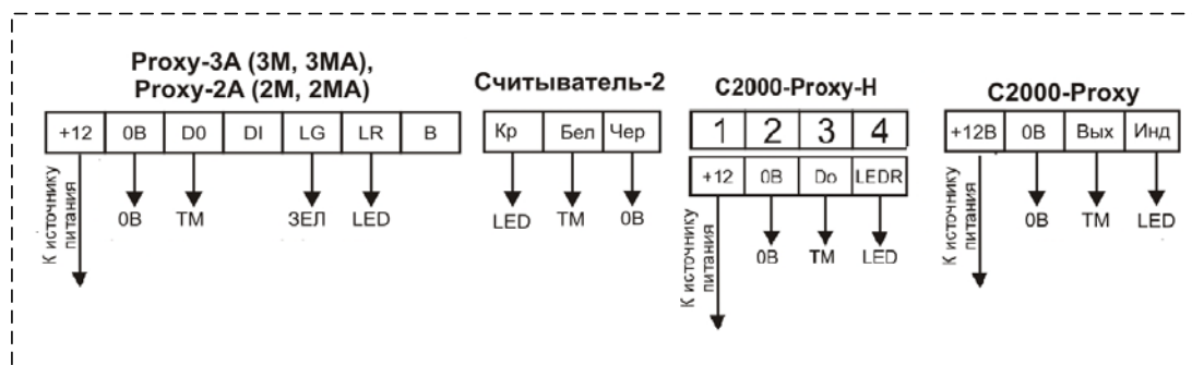
Рисунок 5. Подключение считывателей
