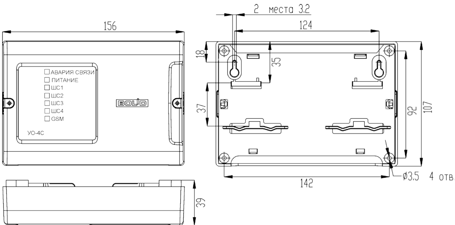
Рисунок 2. Габаритные и установочные размеры
