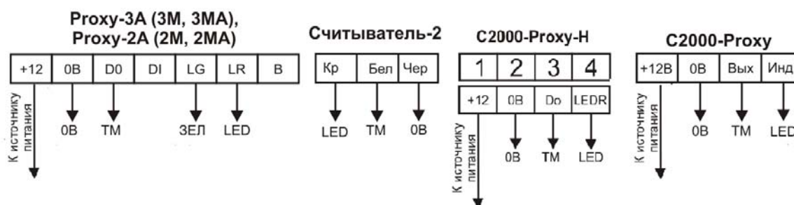
Рисунок 7. Подключение считывателей
